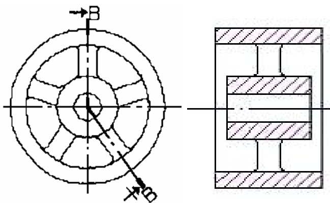
CORTE B-B
