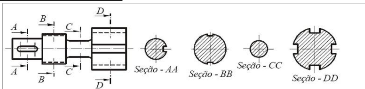
CORTE A-A
