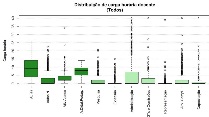
Figura 152 Boxplot Todos
