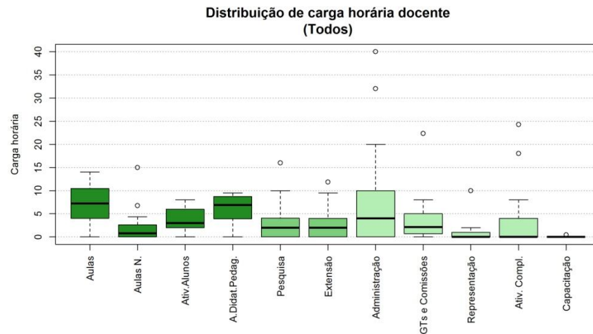
Figura 234 Boxplot Todos
