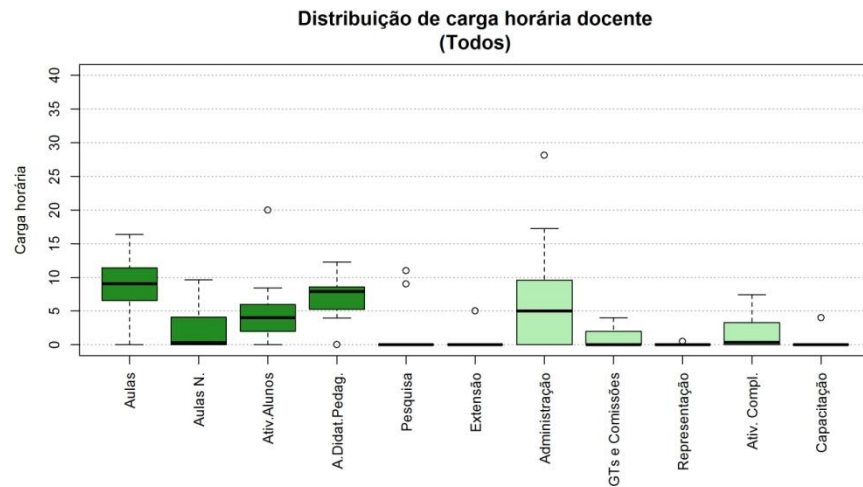
Figura 146 Boxplot Todos
