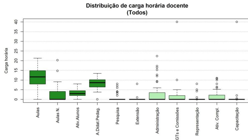
Figura 188 Boxplot Todos
