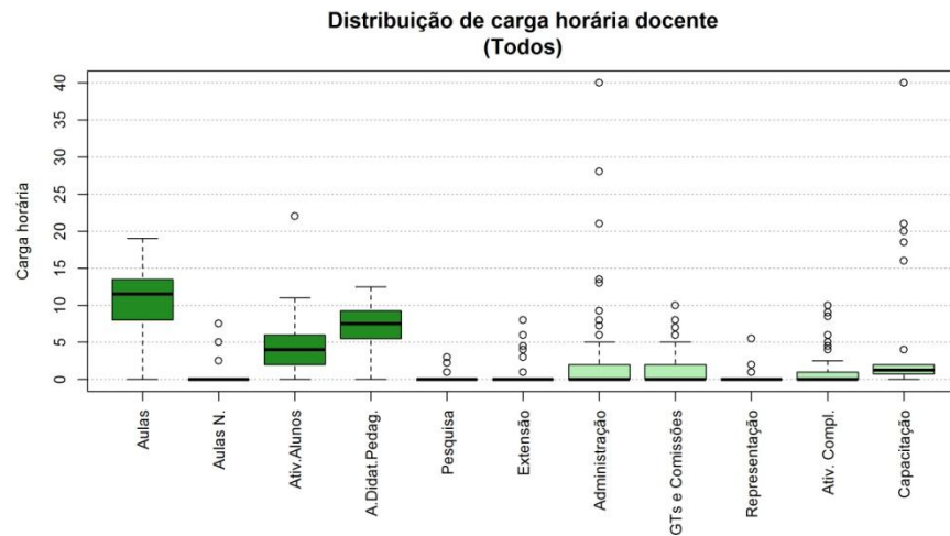
Figura 92 Boxplot Todos
