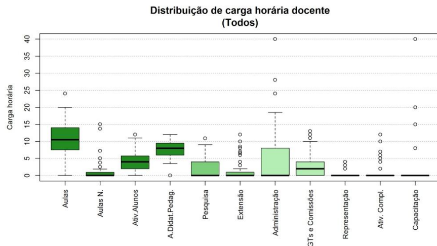
Figura 10 Boxplot Todos
