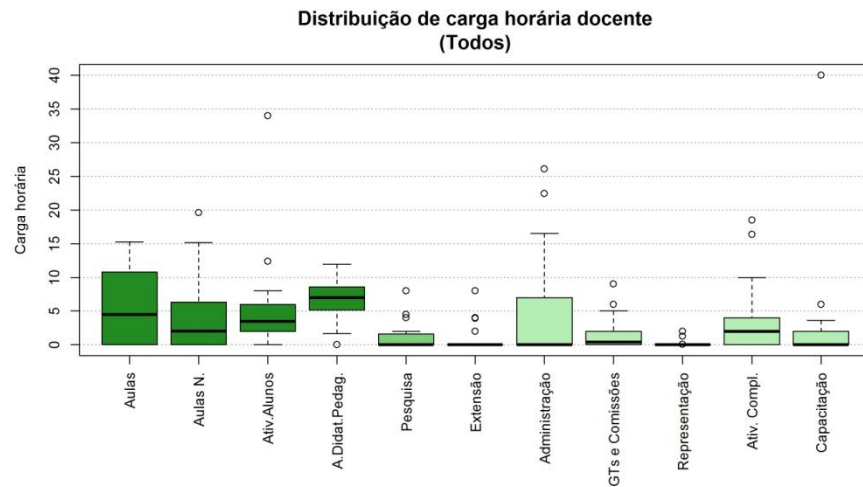
Figura 288 Boxplot Todos
