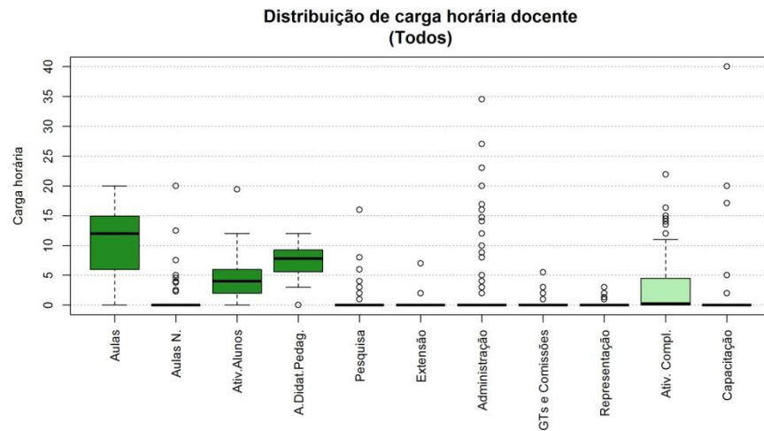
Figura 100 Boxplot Todos
