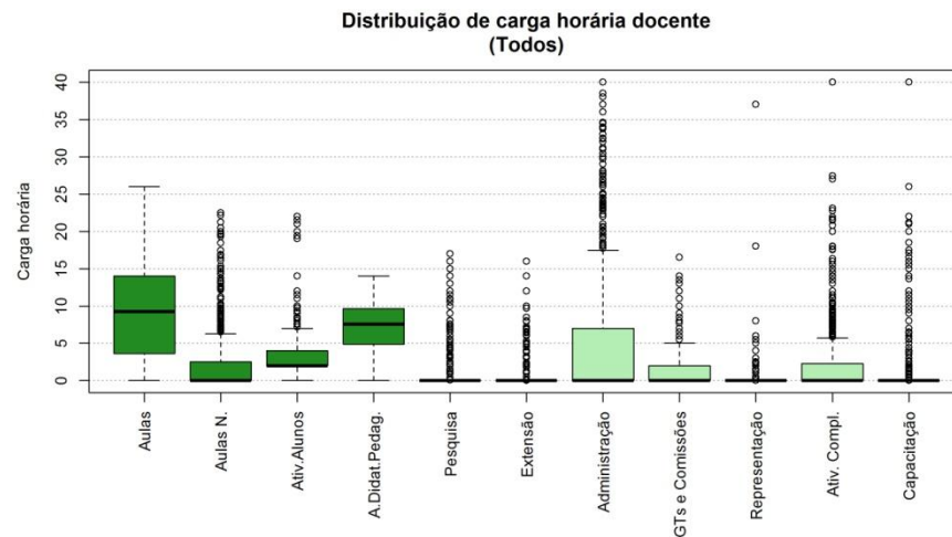
Figura 2 Boxplot Todos
