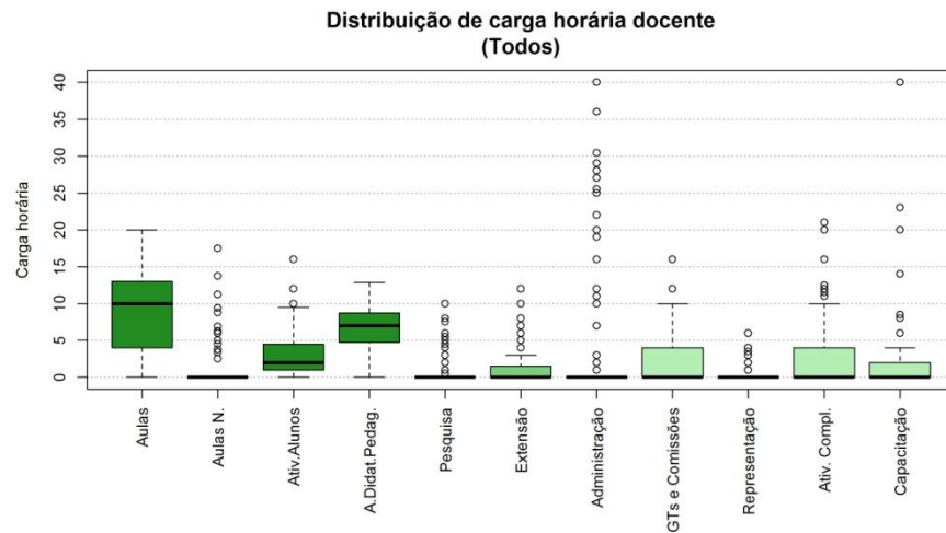
Figura 280 Boxplot Todos
