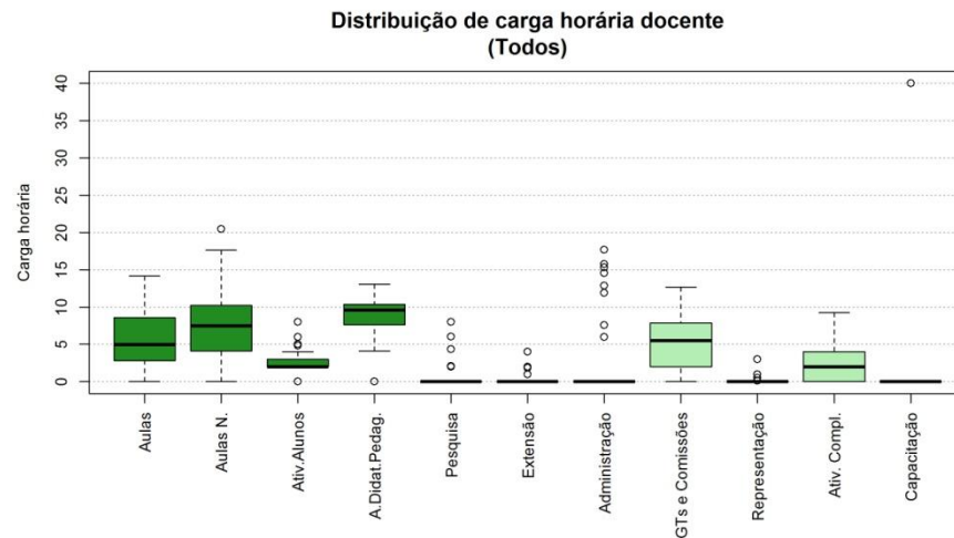
Figura 196 Boxplot Todos
