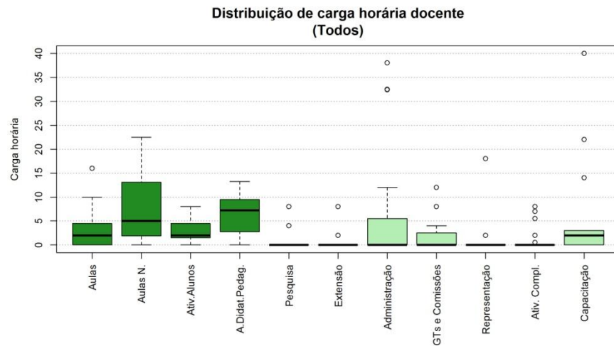
Figura 116 Boxplot Todos
