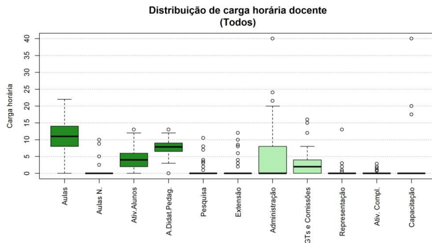
Figura 160 Boxplot Todos
