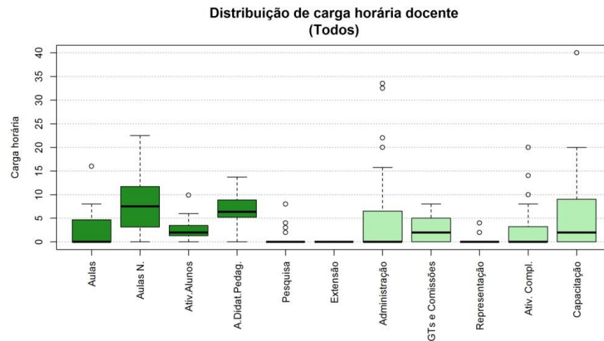
Figura 272 Boxplot Todos
