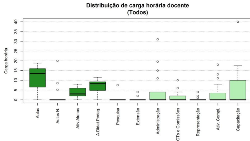
Figura 84 Boxplot Todos
