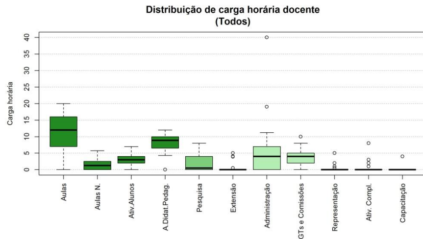
Figura 22 Boxplot Todos
