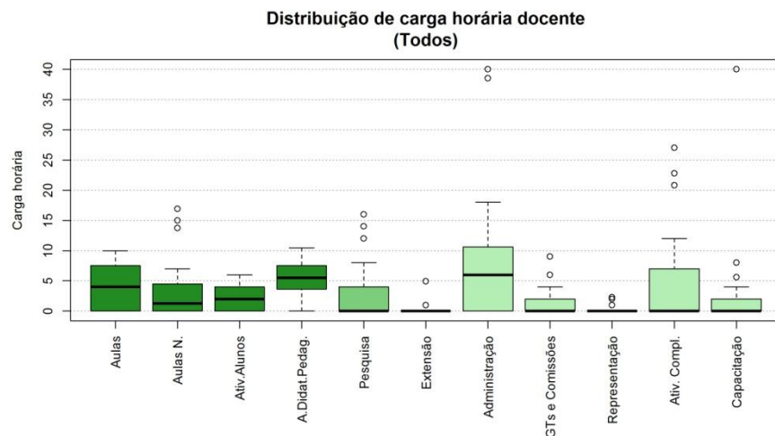
Figura 80 Boxplot Todos
