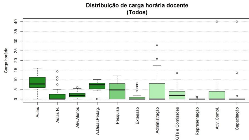
Figura 108 Boxplot Todos
