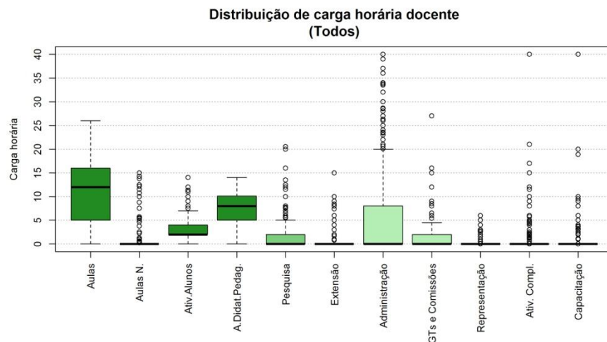
Figura 212 Boxplot Todos
