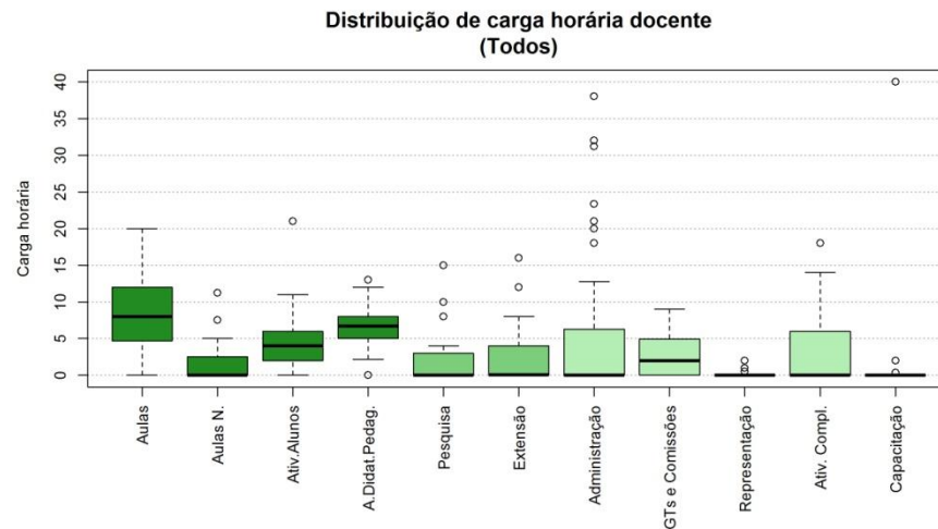
Figura 72 Boxplot Todos
