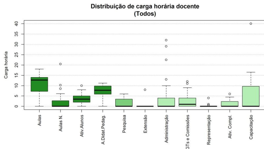
Figura 240 Boxplot Todos
