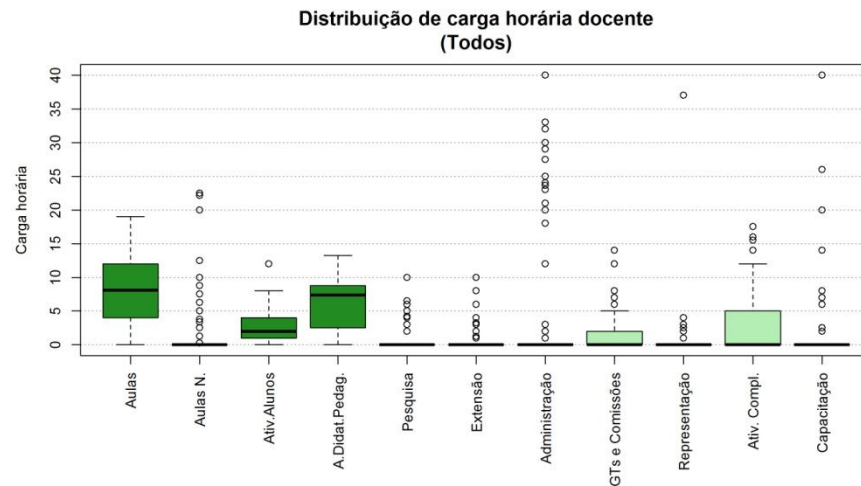
Figura 124 Boxplot Todos
