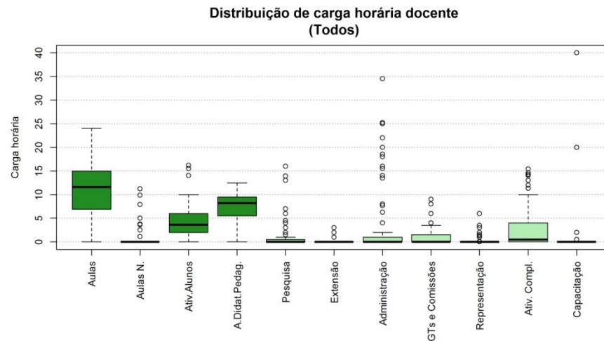
Figura 256 Boxplot Todos
