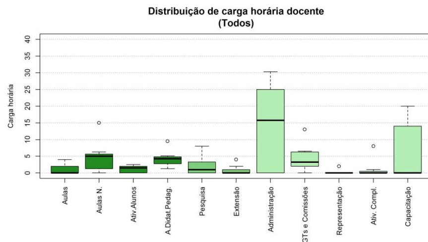
Figura 182 Boxplot Todos
