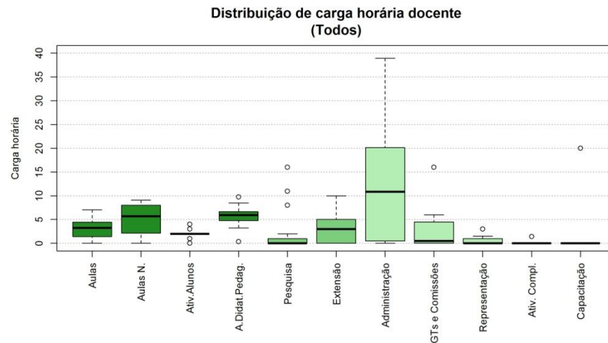
Figura 220 Boxplot Todos
