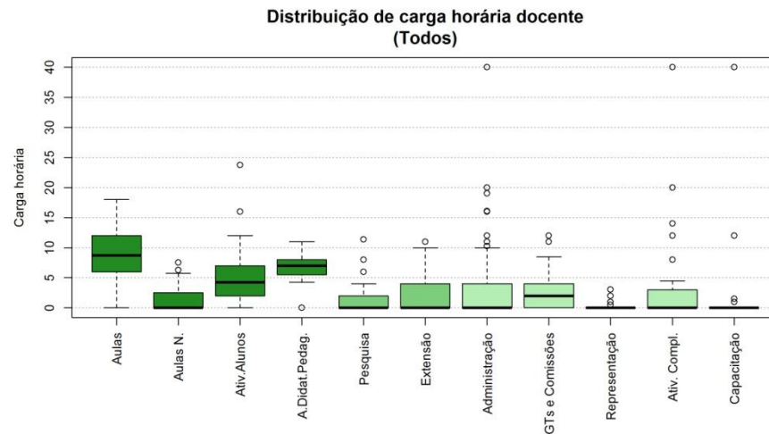
Figura 226 Boxplot Todos
