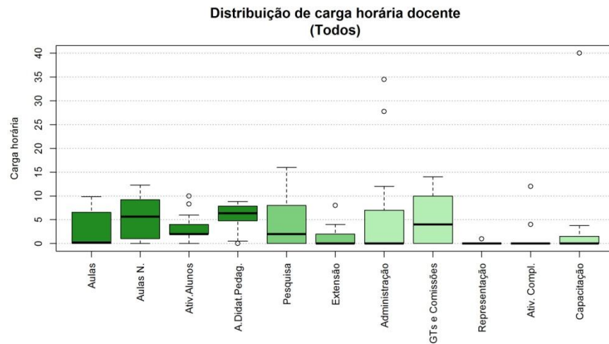
Figura 138 Boxplot Todos
