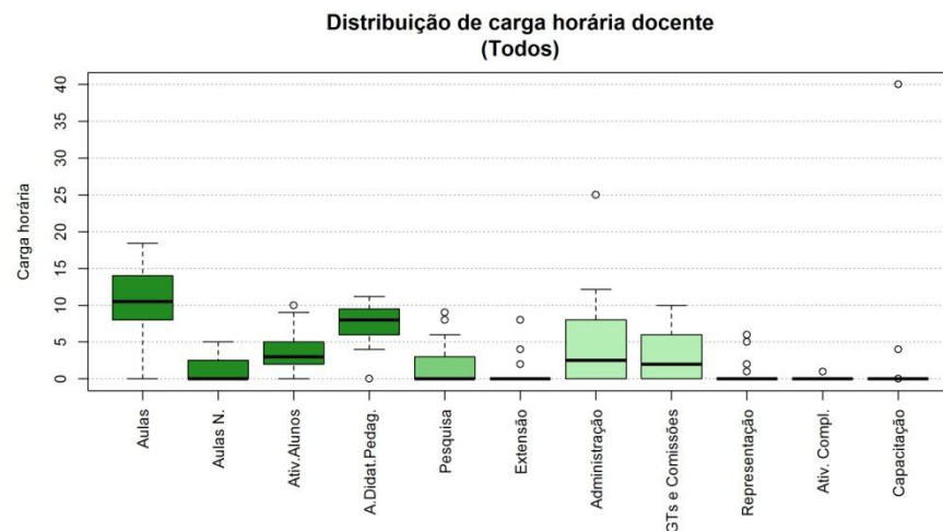
Figura 174 Boxplot Todos
