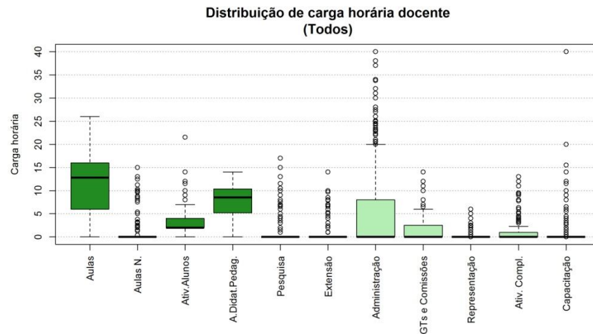
Figura 58 Boxplot Todos
