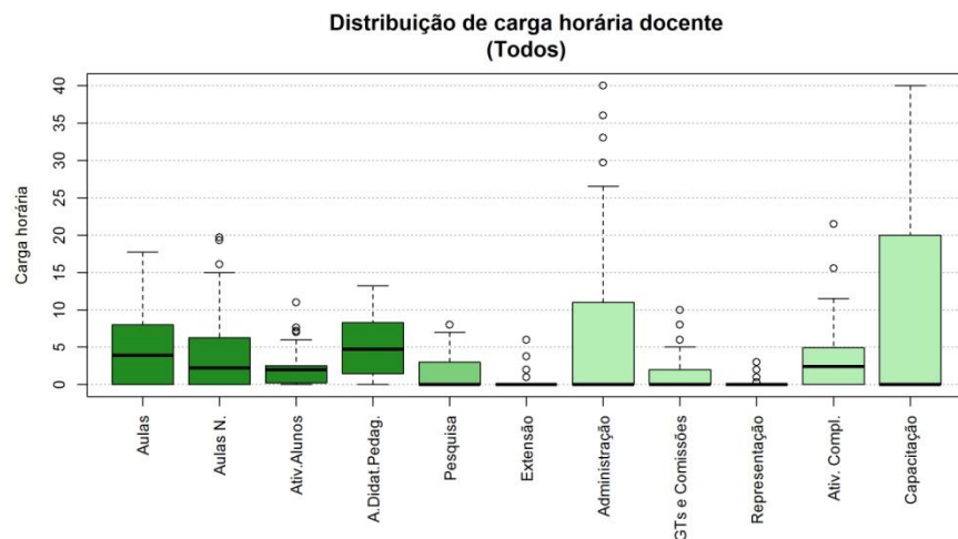
Figura 50 Boxplot Todos
