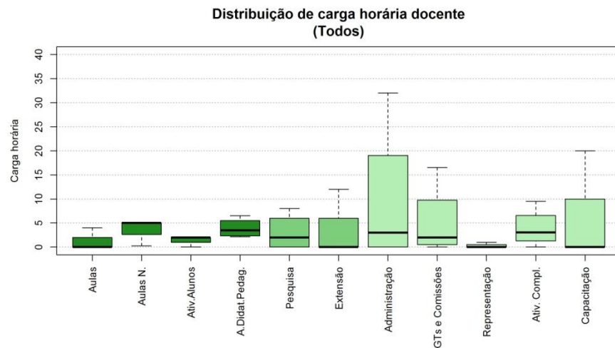
Figura 30 Boxplot Todos
