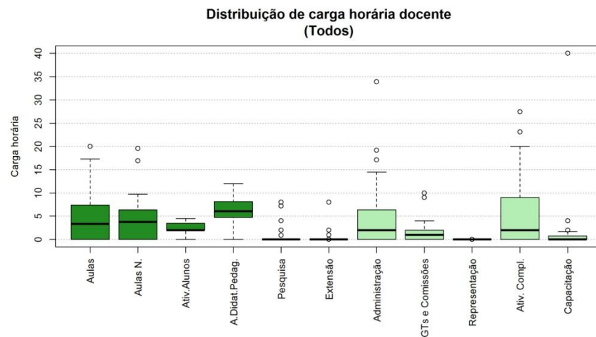
Figura 132 Boxplot Todos
