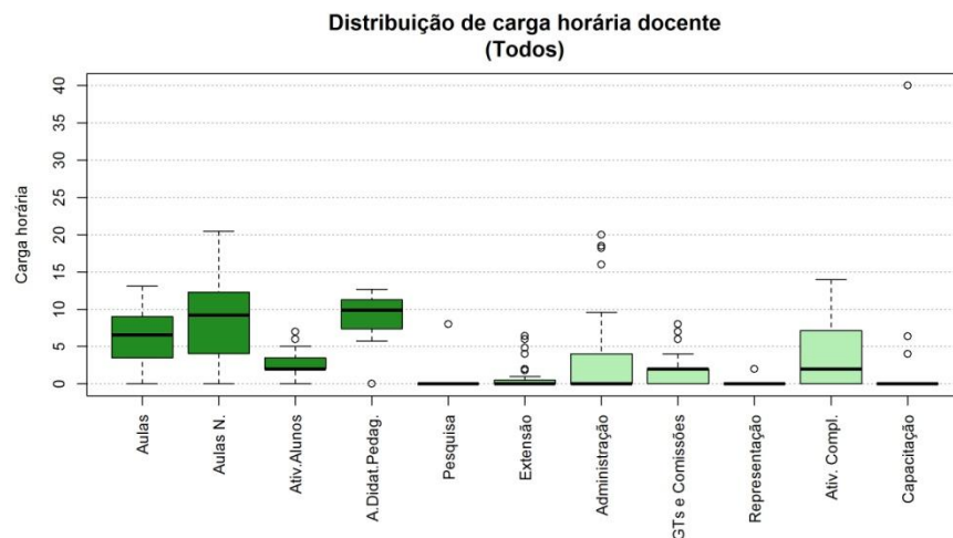
Figura 42 Boxplot Todos
