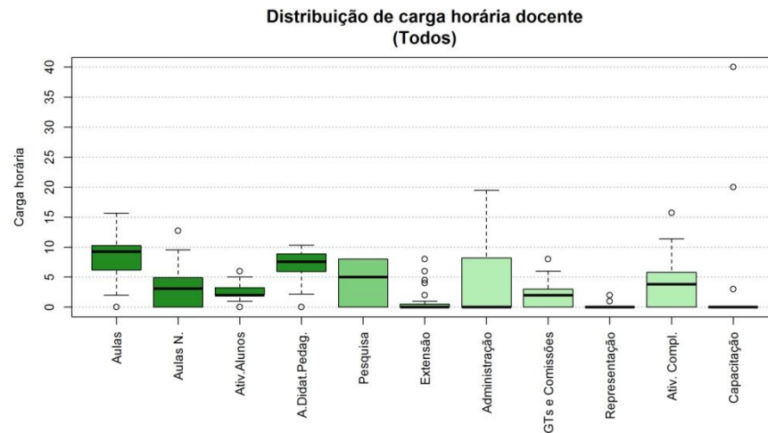
Figura 264 Boxplot Todos
