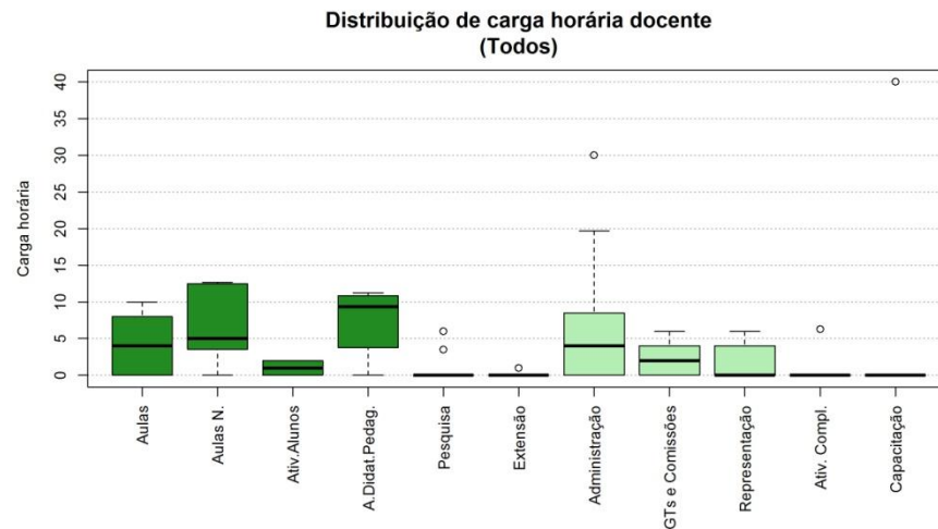
Figura 168 Boxplot Todos
