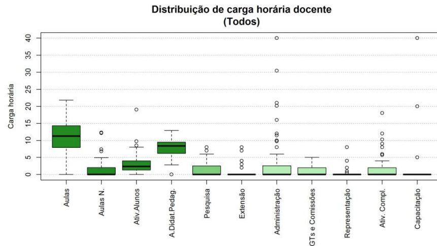
Figura 34 Boxplot Todos
