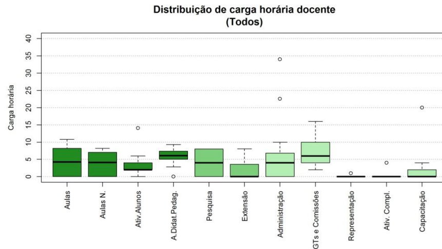
Figura 296 Boxplot Todos
