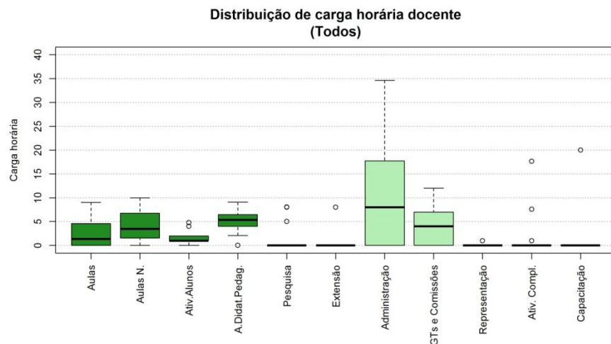
Figura 66 Boxplot Todos
