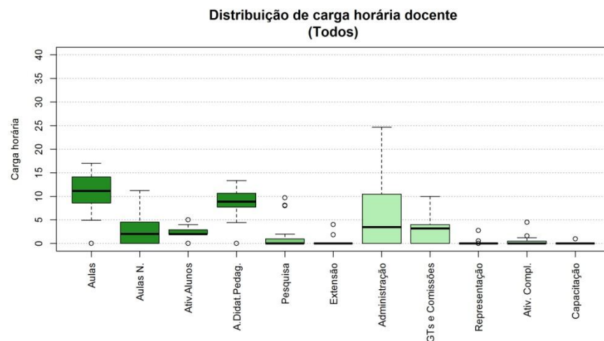
Figura 304 Boxplot Todos
