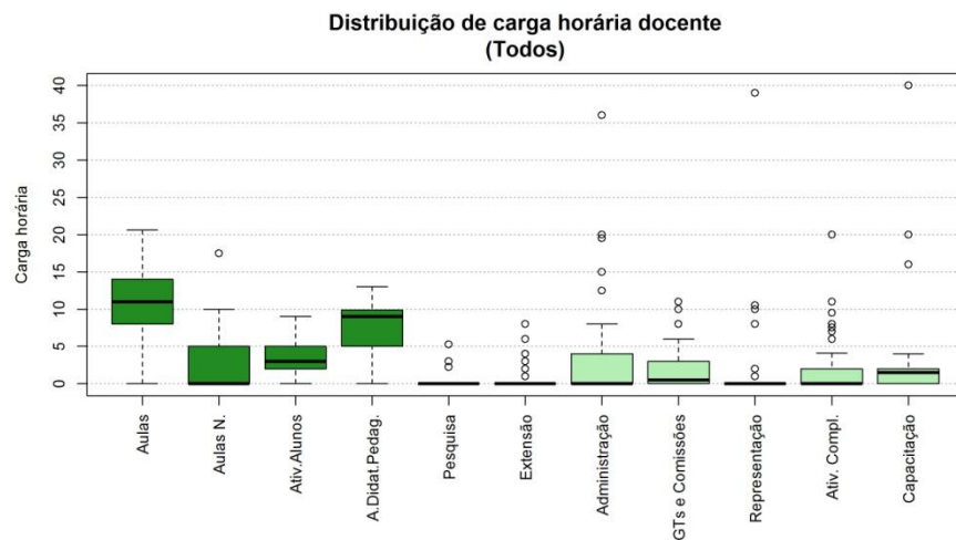
Figura 248 Boxplot Todos
