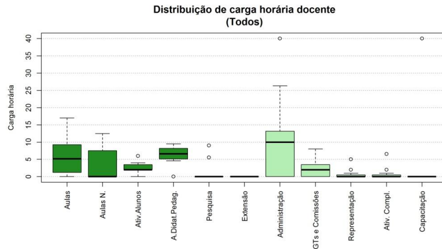
Figura 18 Boxplot Todos
