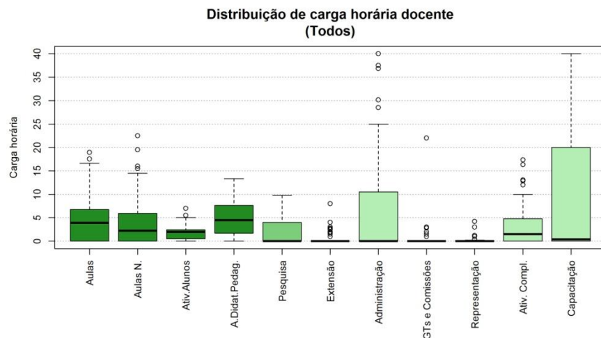
Figura 204 Boxplot Todos
