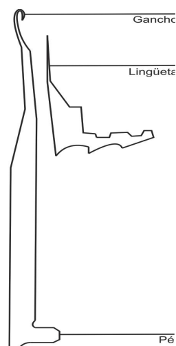
Ilustração 48: Agulha Composta com Ranhura.
