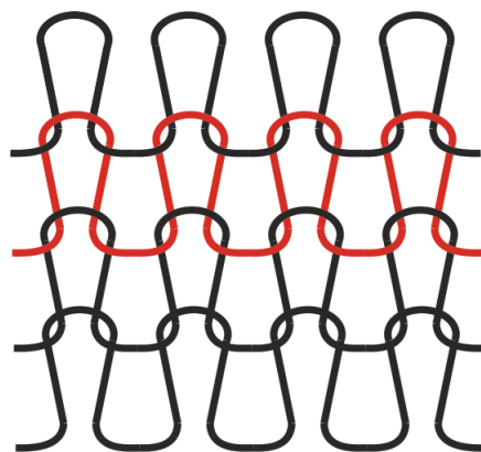
Ilustração 40: Carreira de Malhas (Curso).
