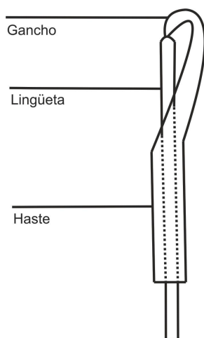
Ilustração 47: Agulha Composta Tubular.
