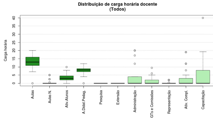
Figura 215 Boxplot Todos
