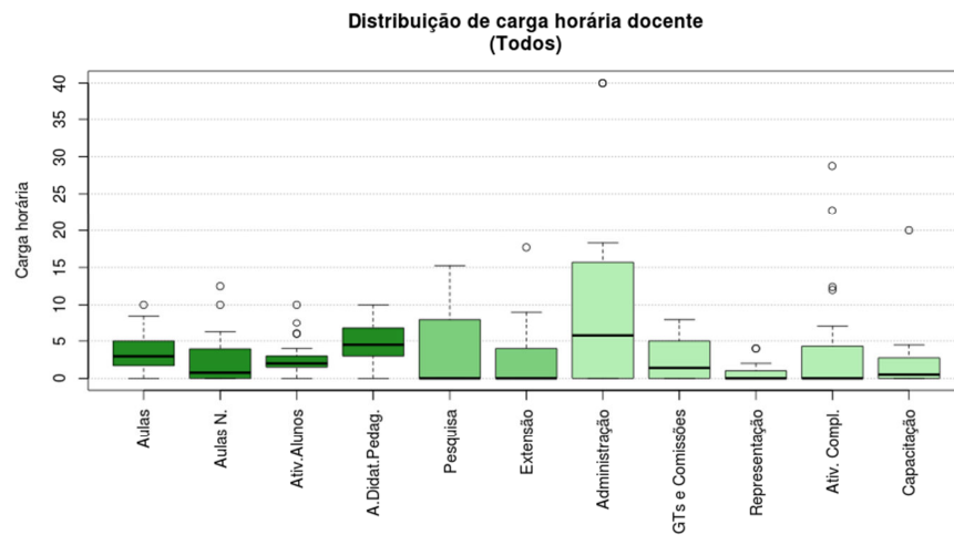
Figura 207 Boxplot Todos
