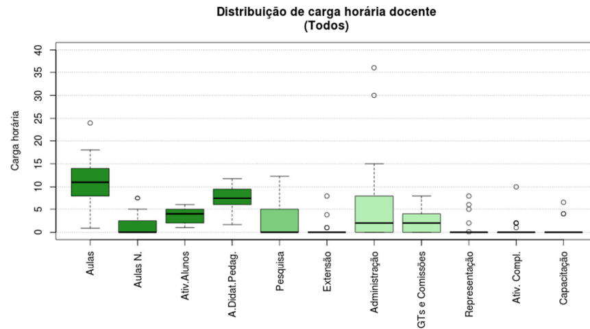
Figura 153 Boxplot Todos
