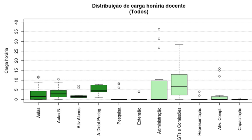
Figura 193 Boxplot Todos
