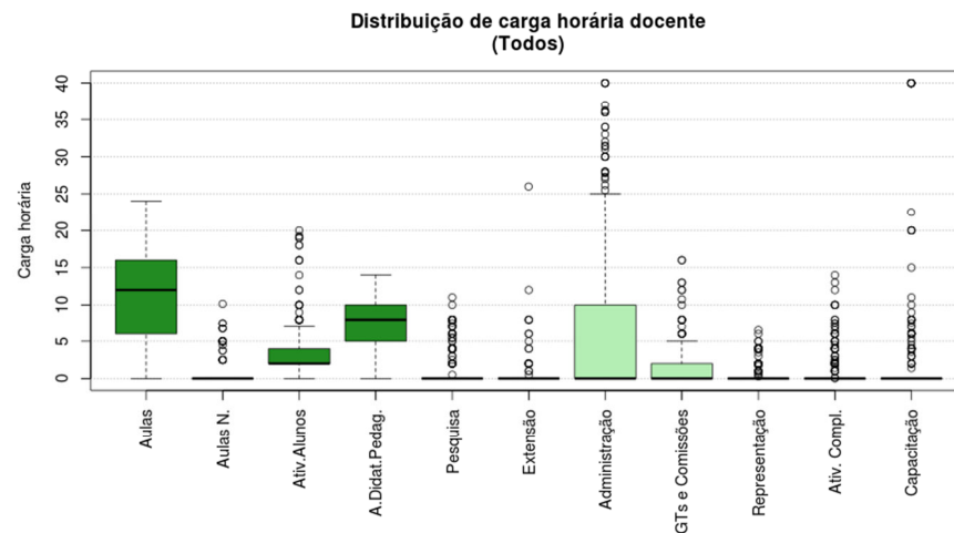
Figura 50 Boxplot Todos
