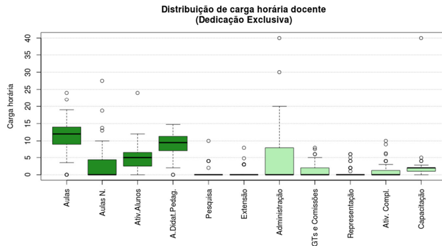
Figura 86 Boxplot Dedicação Exclusiva
