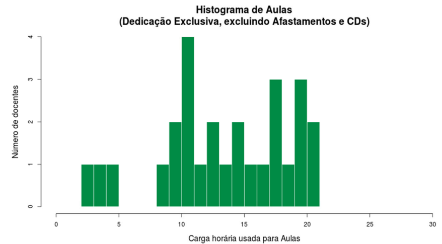
Figura 24 Histograma Aulas Dedicação Exclusiva excl. Afastamentos e CDs
