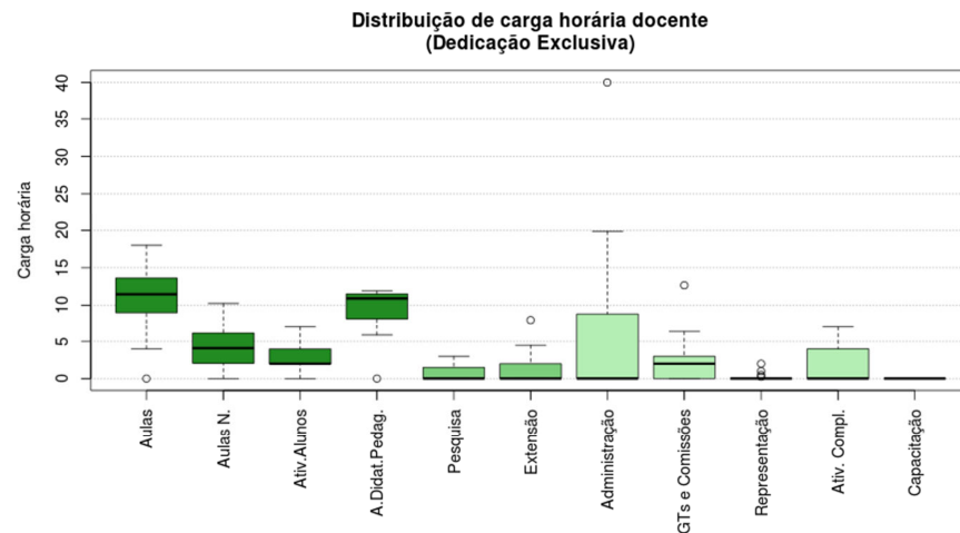
Figura 36 Boxplot Dedicação Exclusiva
