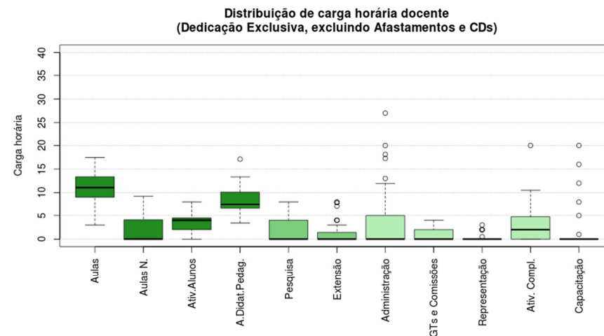
Figura 27 Boxplot Dedicação Exclusiva, excluindo Afastamentos e CDs
