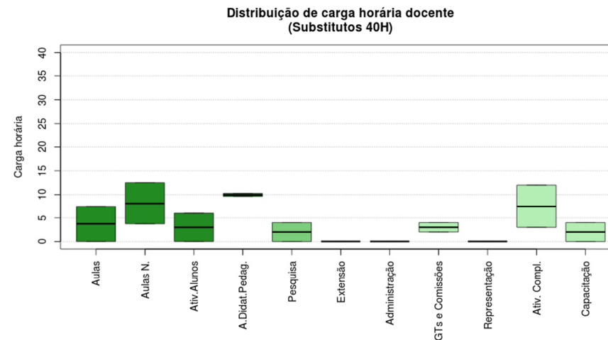
Figura 248 Boxplot Substitutos 40H
