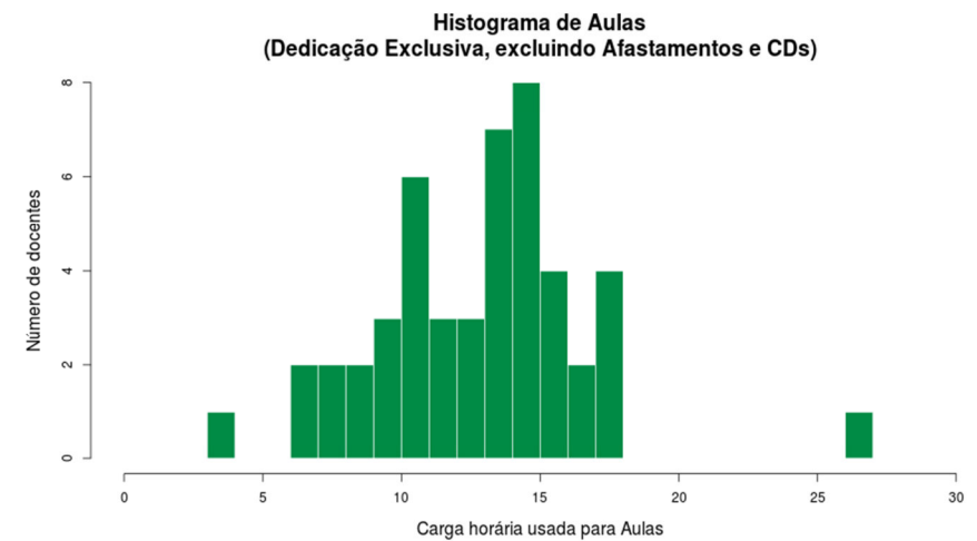
Figura 32 Histograma Aulas Dedicação Exclusiva excl. Afastamentos e CDs
