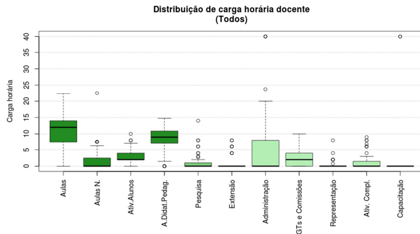
Figura 10 Boxplot Todos
