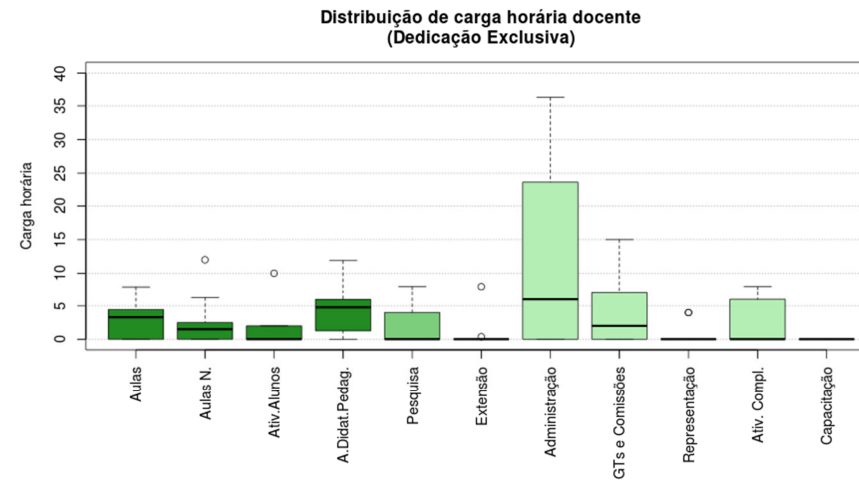
Figura 60 Boxplot Dedicação Exclusiva
