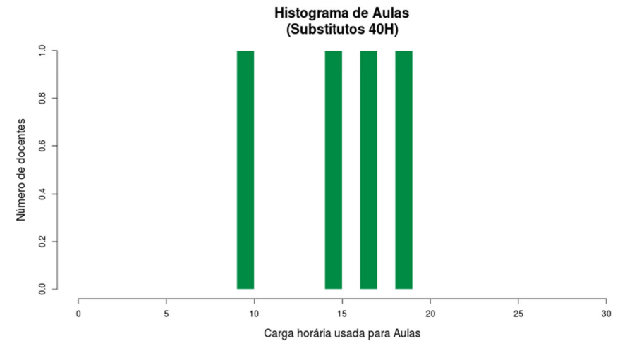
Figura 206 Histograma Aulas Substitutos 40H
