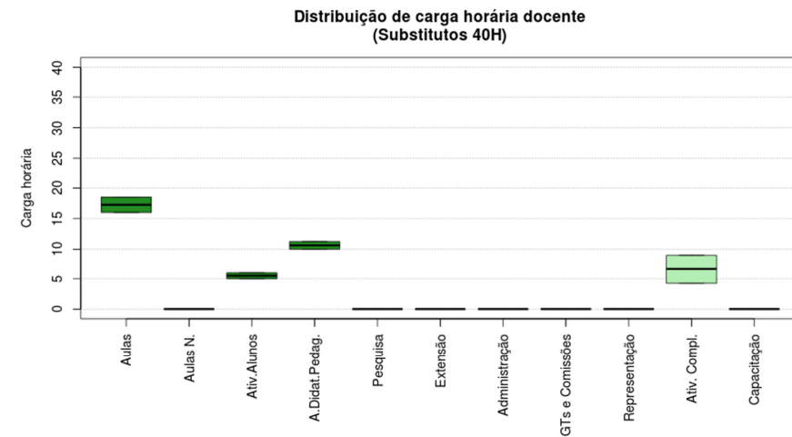
Figura 67 Boxplot Substitutos 40H
