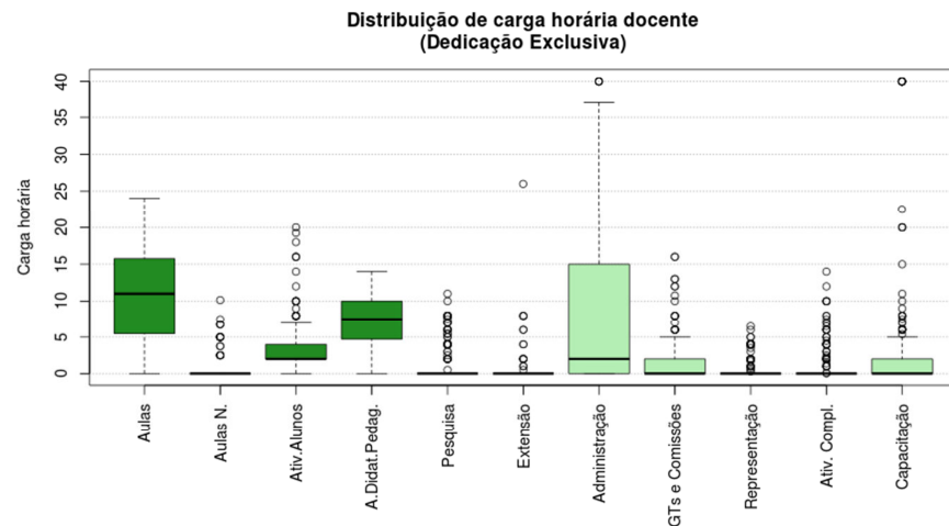
Figura 52 Boxplot Dedicação Exclusiva
