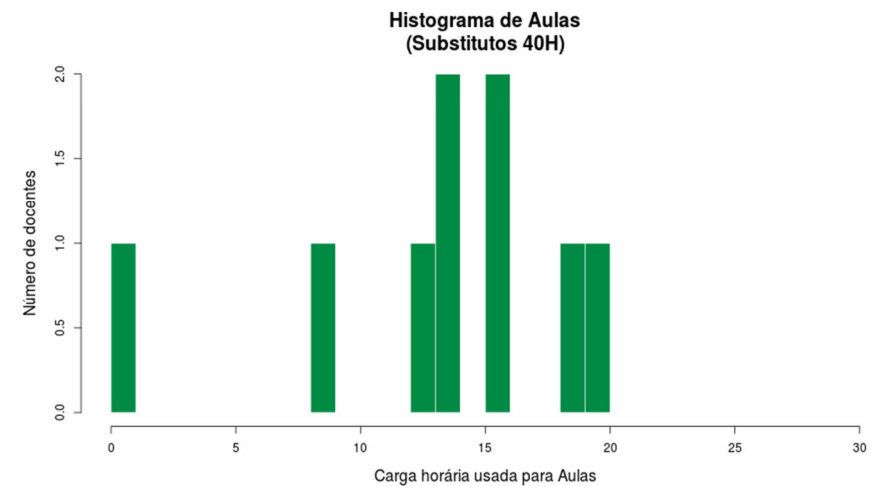
Figura 122 Histograma Aulas Substitutos 40H
