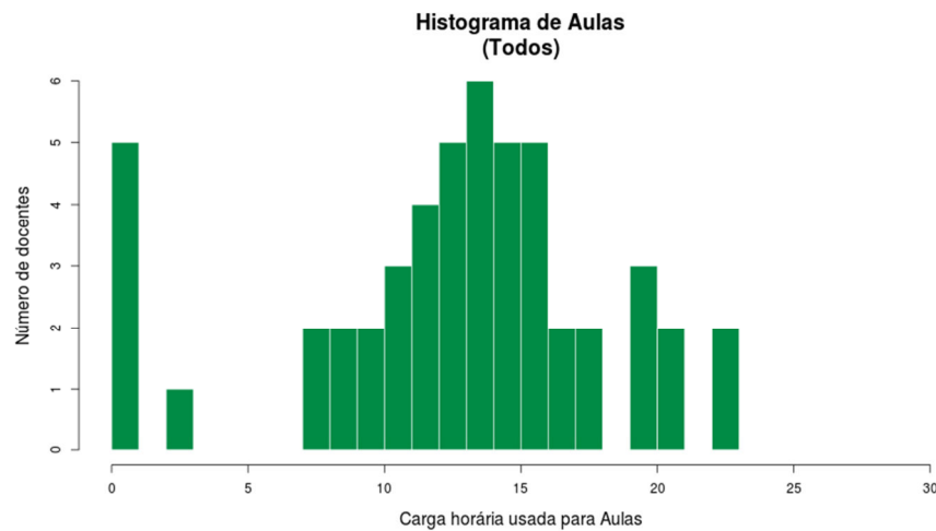
Figura 14 Histograma Aulas Todos
