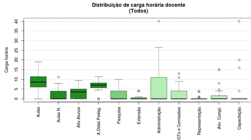
Figura 199 Boxplot Todos
