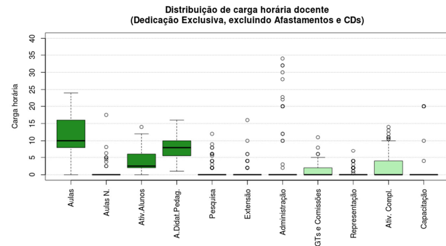
Figura 254 Boxplot Dedicação Exclusiva, excluindo Afastamentos e CDs
