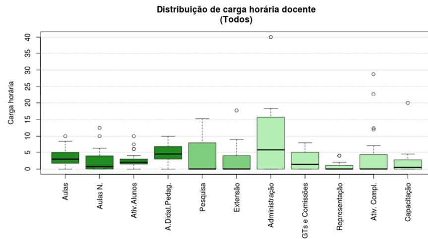
Figura 207 Boxplot Todos
