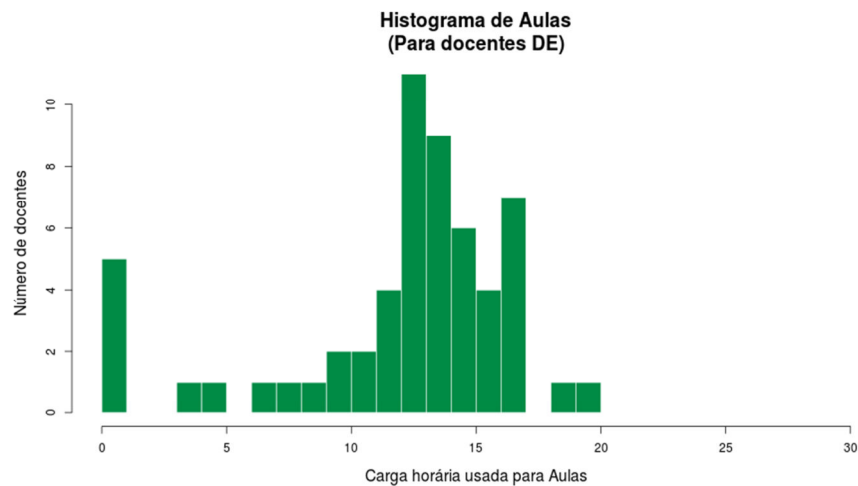
Figura 236 Histograma Aulas Dedicação Exclusiva
