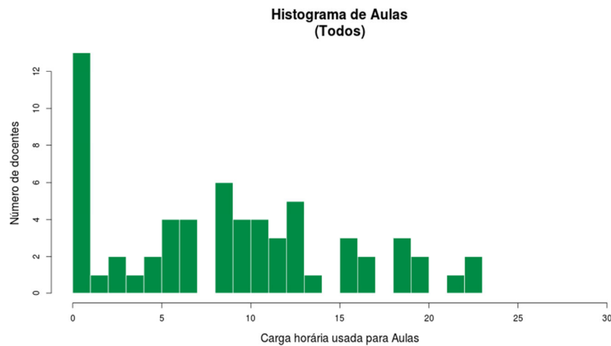
Figura 181 Histograma Aulas Todos
