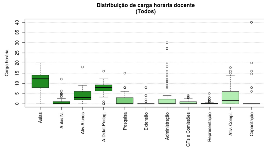
Figura 231 Boxplot Todos
