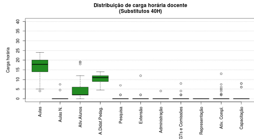
Figura 53 Boxplot Substitutos 40H
