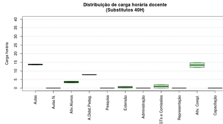
Figura 241 Boxplot Substitutos 40H
