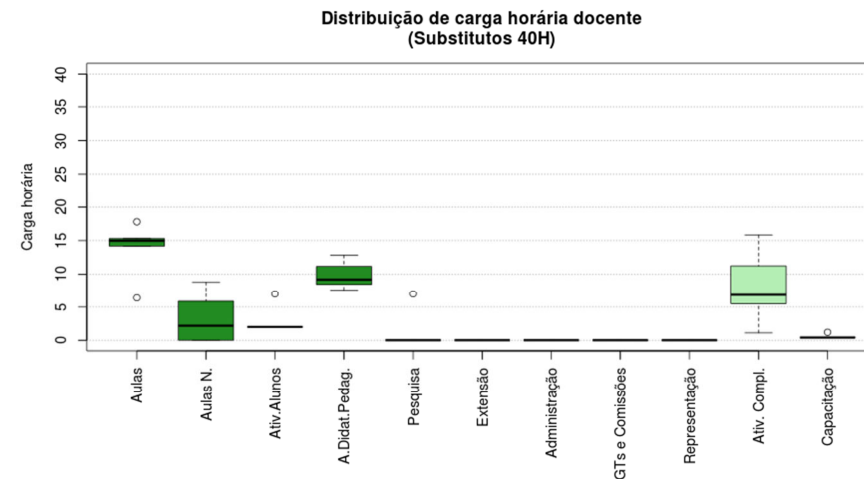
Figura 45 Boxplot Substitutos 40H
