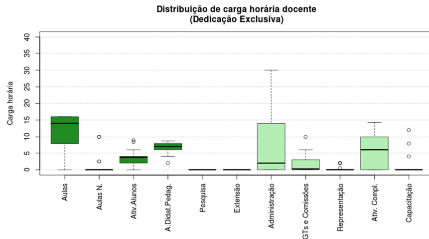
Figura 78 Boxplot Dedicação Exclusiva
