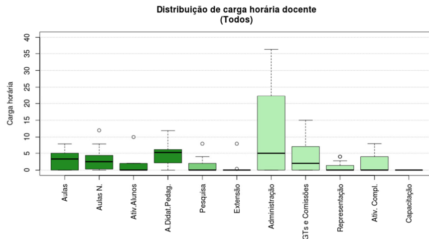
Figura 58 Boxplot Todos
