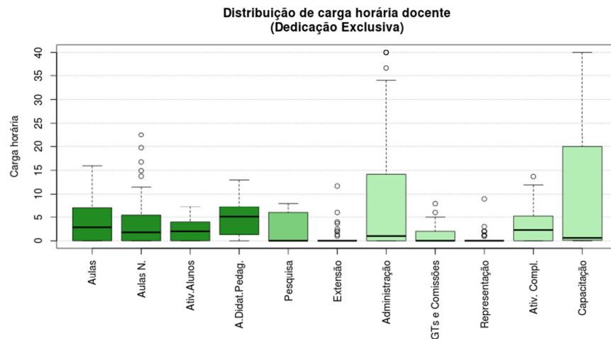
Figura 179 Boxplot Dedicação Exclusiva
