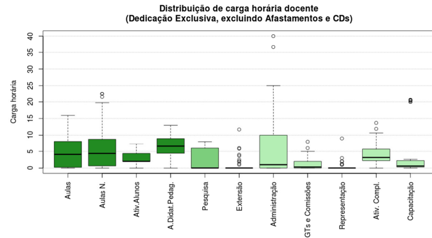
Figura 178 Boxplot Dedicação Exclusiva, excluindo Afastamentos e CDs
