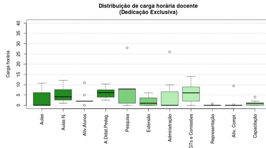
Figura 273 Boxplot Dedicação Exclusiva
