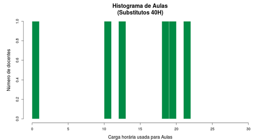
Figura 91 Histograma Aulas Substitutos 40H
