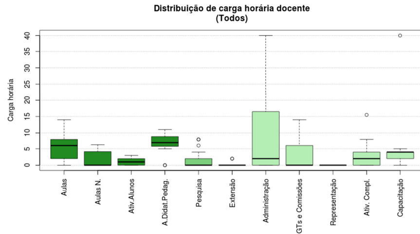
Figura 107 Boxplot Todos
