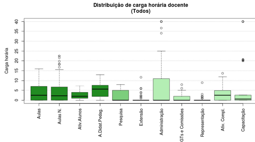
Figura 177 Boxplot Todos
