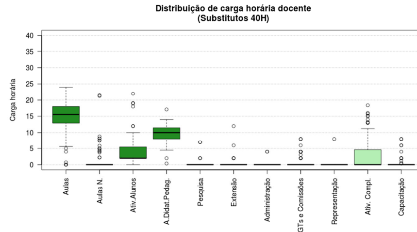
Figura 22 Boxplot Substitutos 40H
