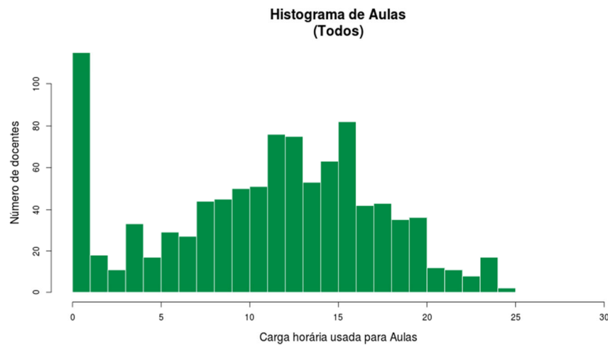
Figura 137 Histograma Aulas Todos
