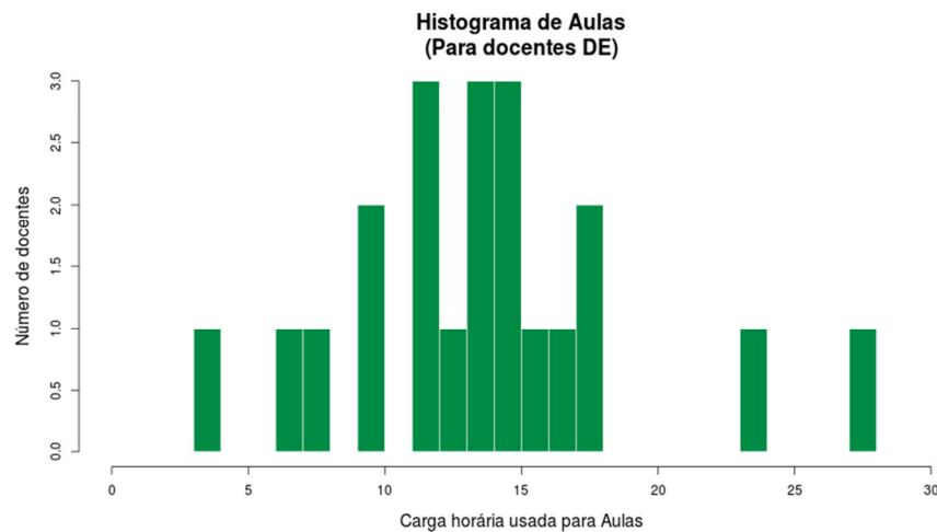
Figura 69 Histograma Aulas Dedicação Exclusiva
