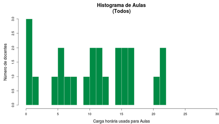
Figura 264 Histograma Aulas Todos
