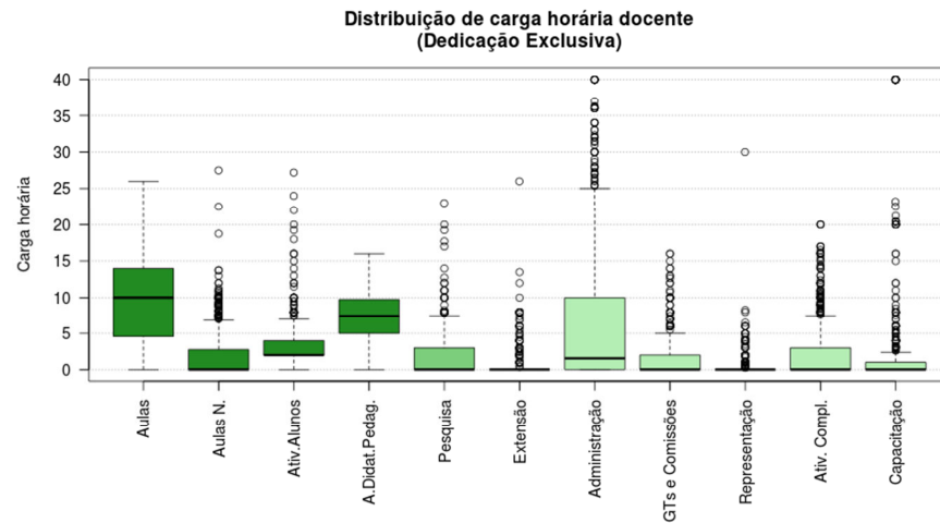
Figura 4 Boxplot Dedicação Exclusiva
