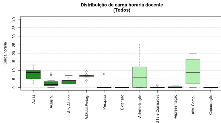
Figura 18 Boxplot Todos
