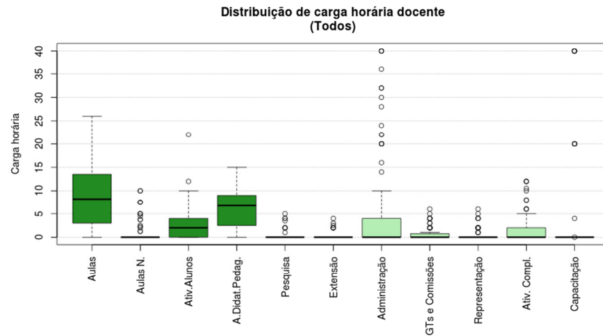
Figura 115 Boxplot Todos
