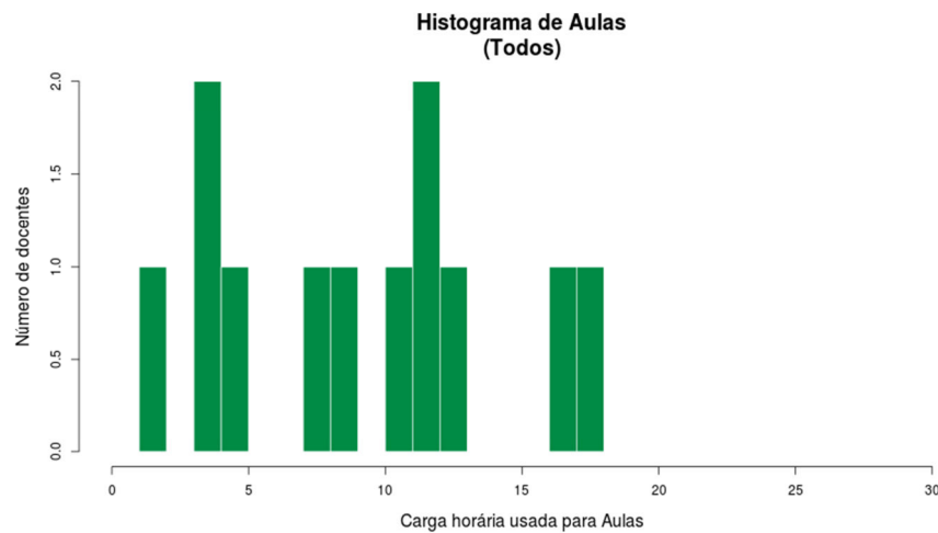
Figura 269 Histograma Aulas Todos
