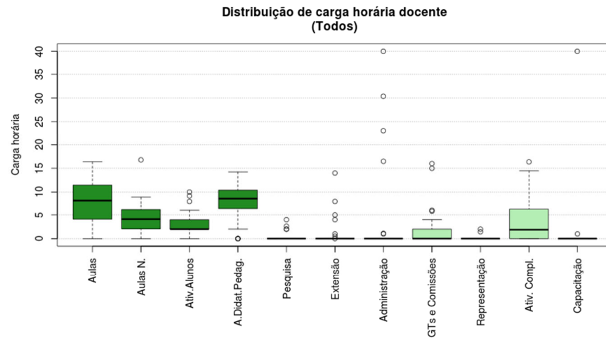
Figura 169 Boxplot Todos
