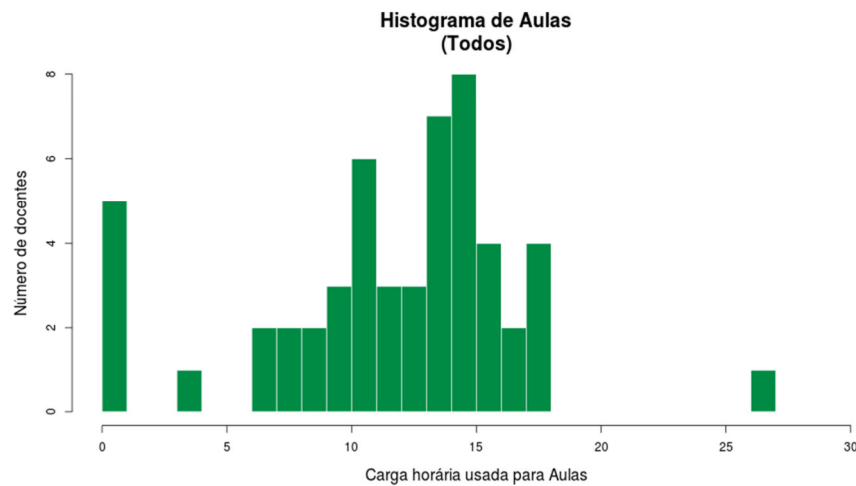
Figura 30 Histograma Aulas Todos
