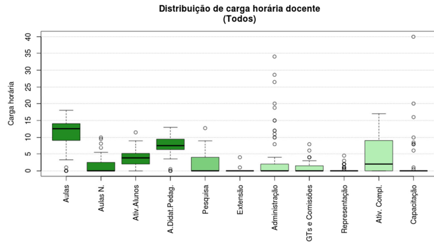
Figura 92 Boxplot Todos
