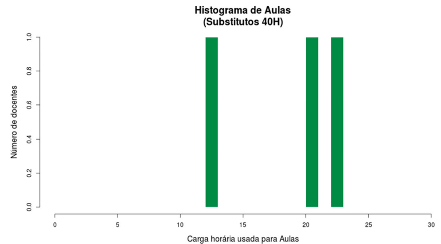
Figura 106 Histograma Aulas Substitutos 40H
