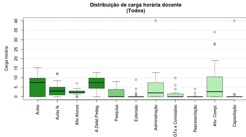
Figura 261 Boxplot Todos
