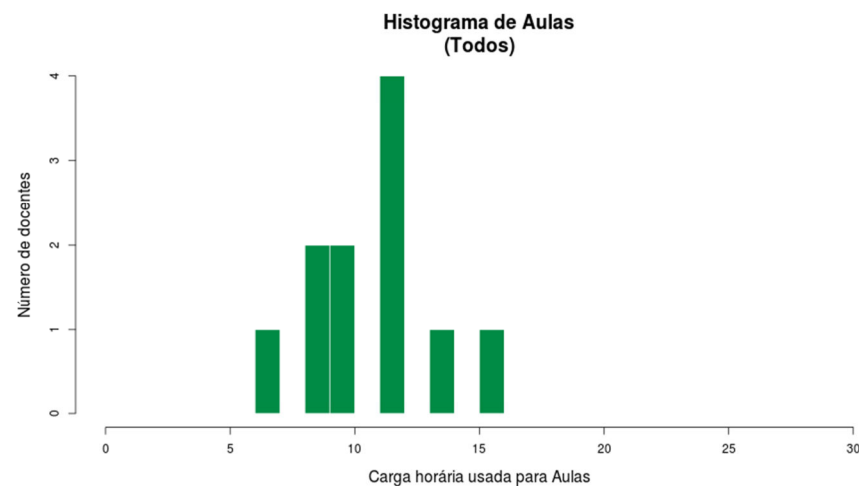
Figura 19 Histograma Aulas Todos
