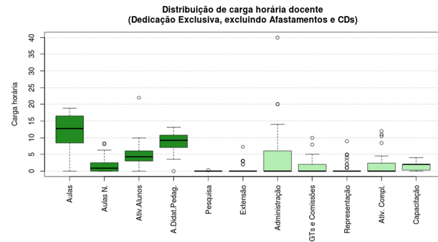
Figura 224 Boxplot Dedicação Exclusiva, excluindo Afastamentos e CDs
