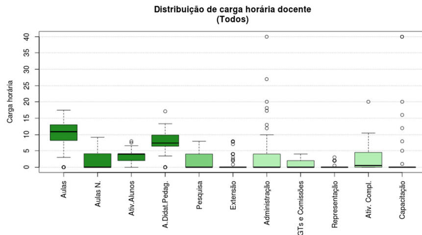
Figura 26 Boxplot Todos
