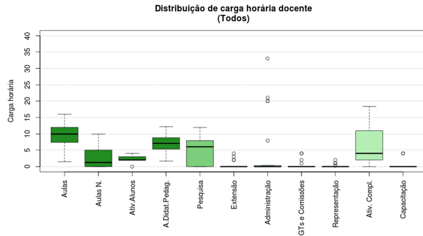
Figura 100 Boxplot Todos
