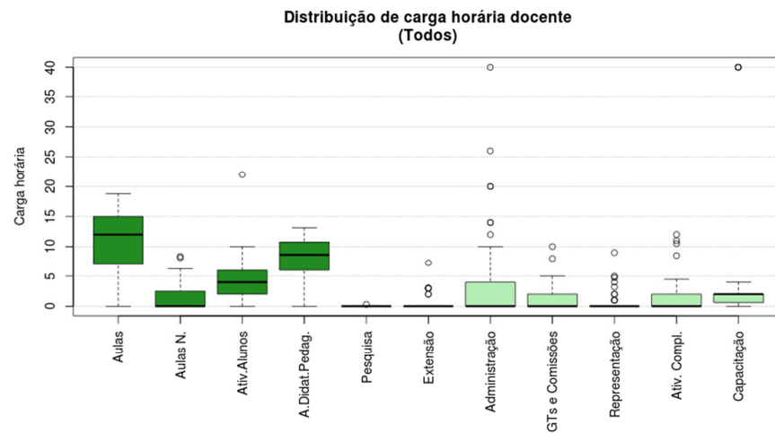
Figura 223 Boxplot Todos
