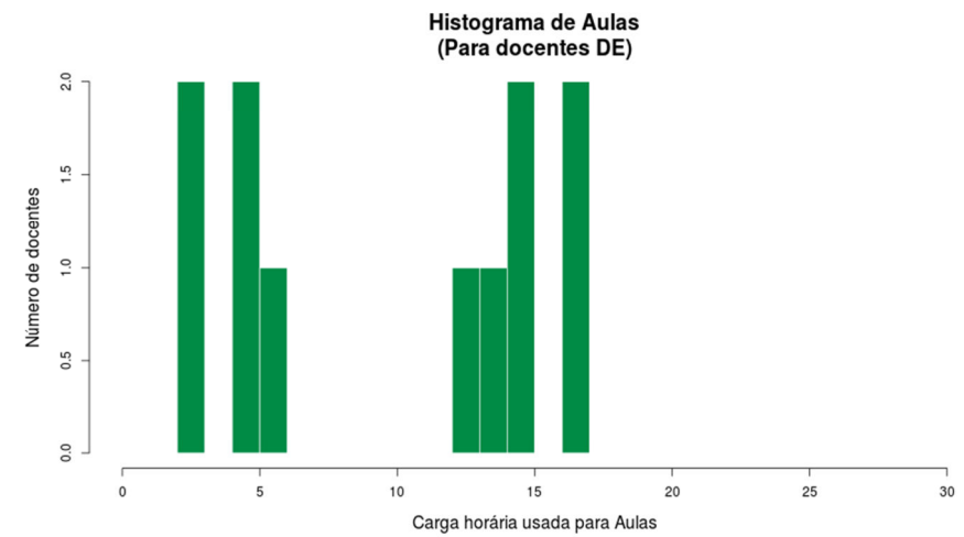
Figura 129 Histograma Aulas Dedicção Exclusiva excl. Afastamentos e CDs
