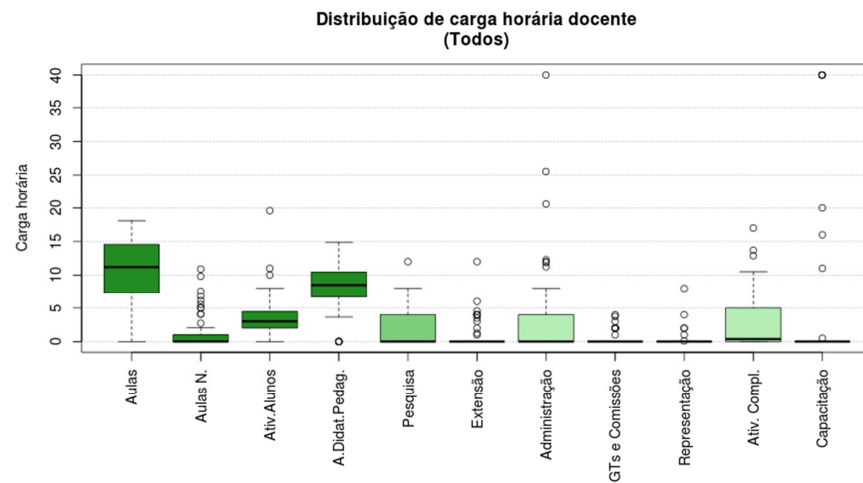
Figura 161 Boxplot Todos
