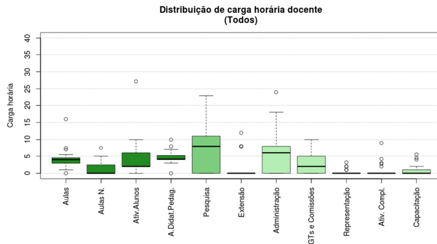
Figura 72 Boxplot Todos
