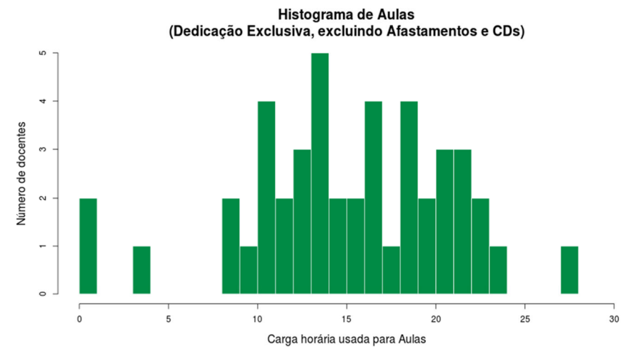
Figura 90 Histograma Aulas Dedicação Exclusiva excl. Afastamentos e CDs
