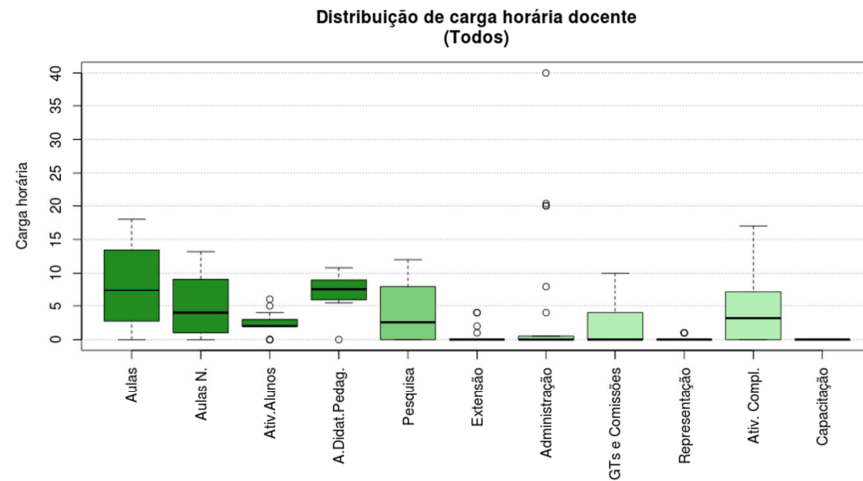
Figura 239 Boxplot Todos
