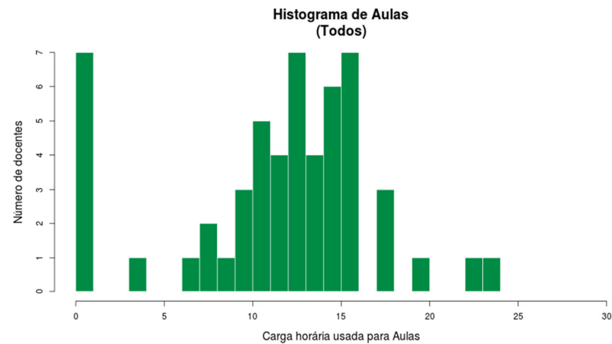
Figura 165 Histograma Aulas Todos
