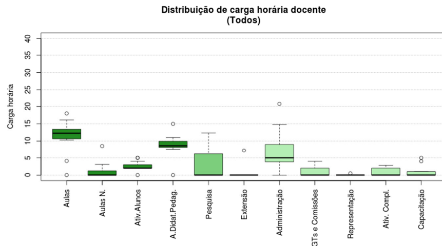
Figura 272 Boxplot Todos
