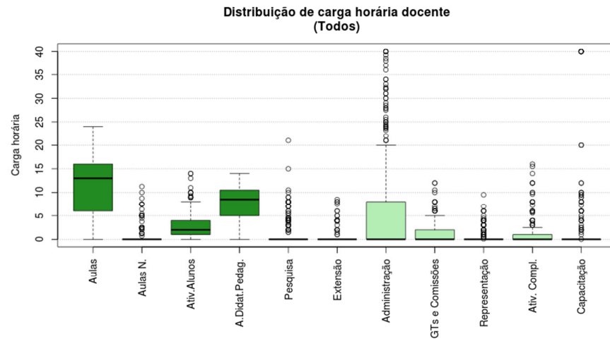
Figura 185 Boxplot Todos
