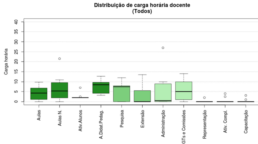
Figura 125 Boxplot Todos
