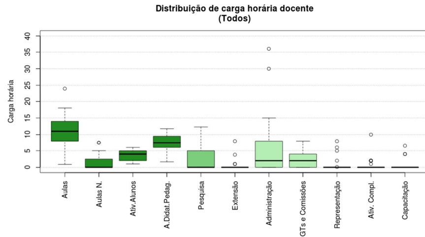
Figura 153 Boxplot Todos
