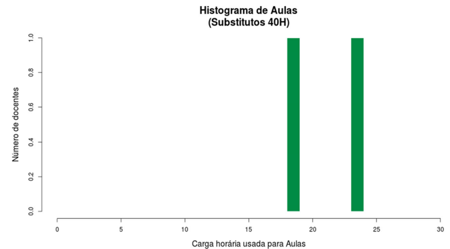
Figura 41 Histograma Aulas Substitutos 40H
