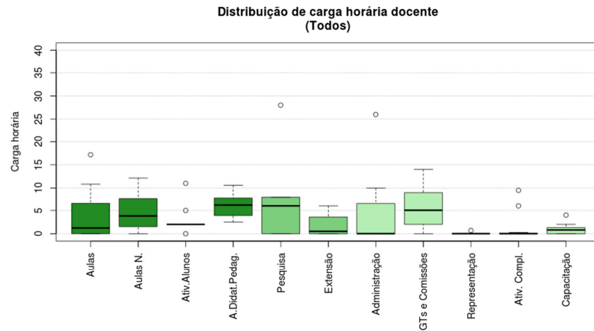
Figura 267 Boxplot Todos
