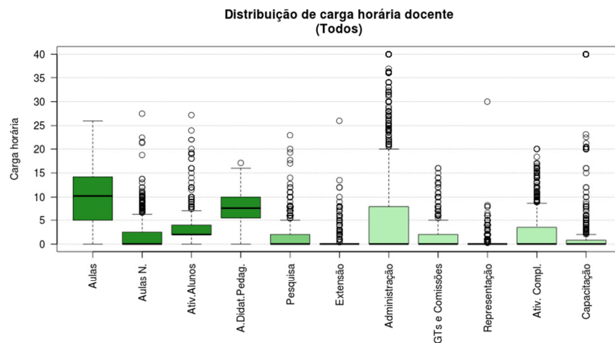
Figura 2 Boxplot Todos
