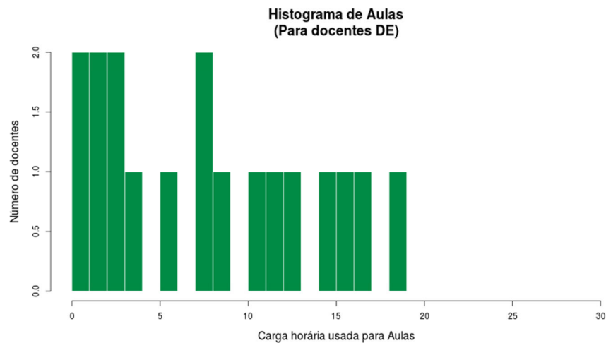
Figura 250 Histograma Aulas Dedicação Exclusiva
