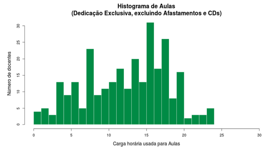
Figura 56 Histograma Aulas Dedicação Exclusiva excl. Afastamentos e CDs
