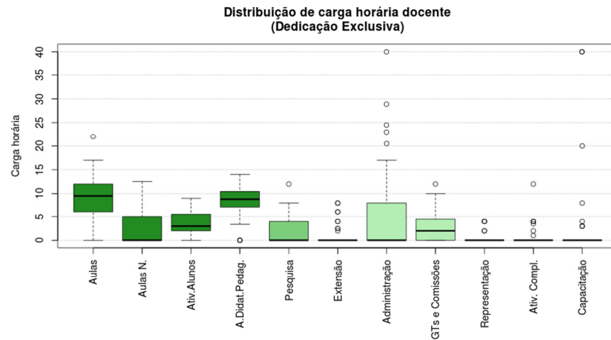
Figura 143 Boxplot Dedicação Exclusiva
