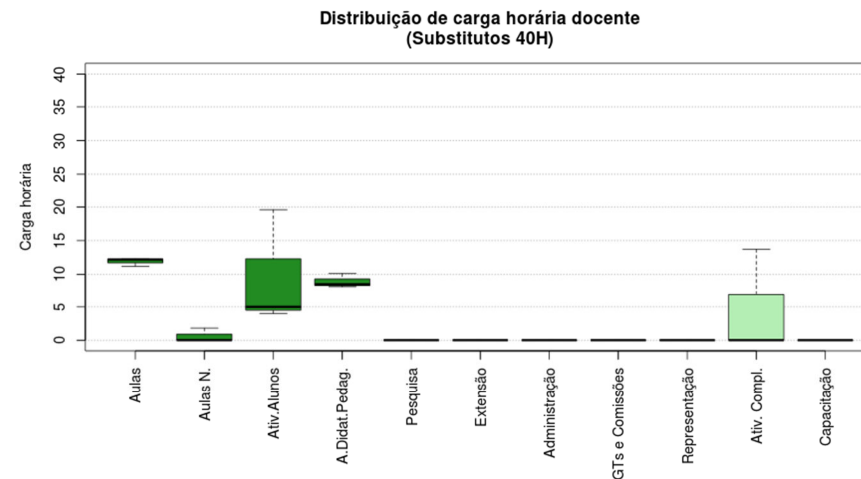
Figura 164 Boxplot Substitutos 40H
