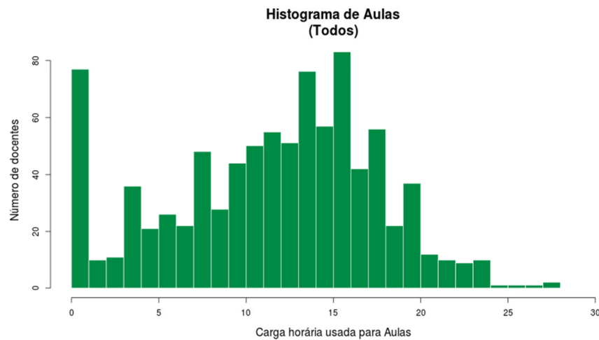
Figura 6 Histograma Aulas Todos
