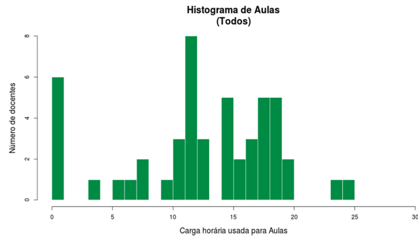
Figura 227 Histograma Aulas Todos
