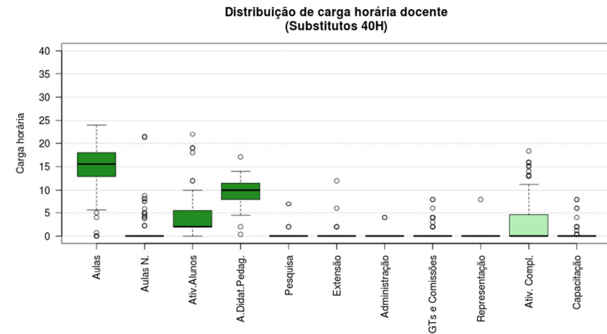
Figura 5 Boxplot Substitutos 40H
