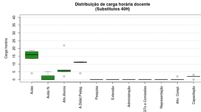
Figura 226 Boxplot Substitutos 40H
