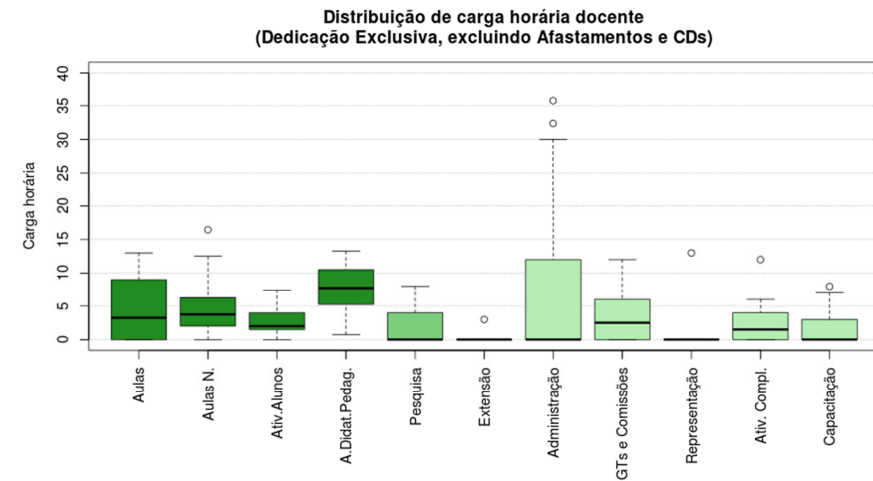
Figura 246 Boxplot Dedicação Exclusiva, excluindo Afastamentos e CDs
