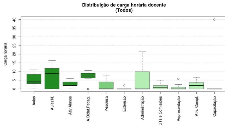
Figura 149 Boxplot Todos
