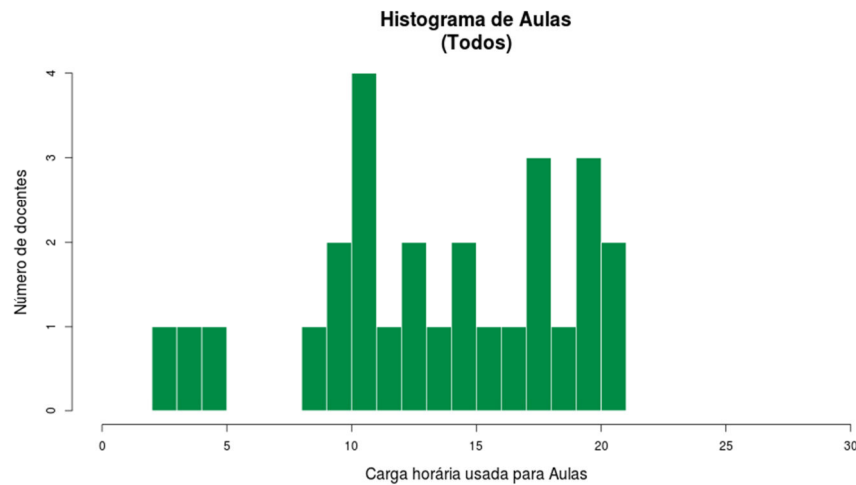
Figura 23 Histograma Aulas Todos
