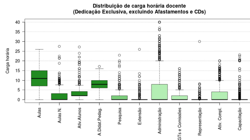
Figura 3 Boxplot Dedicação Exclusiva, excluindo Afastamentos e CDs
