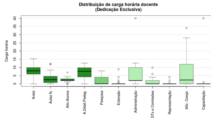
Figura 263 Boxplot Todos
