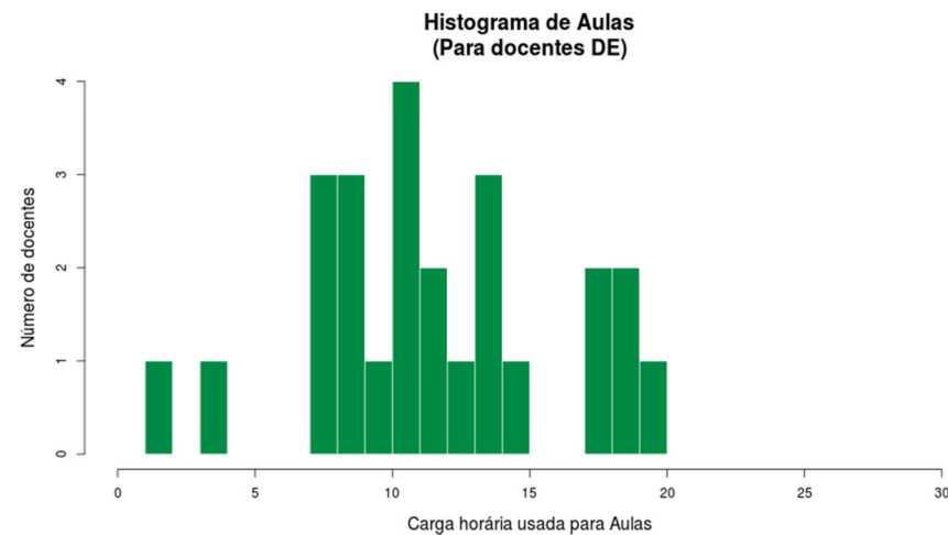
Figura 158 Histograma Aulas Dedicação Exclusiva
