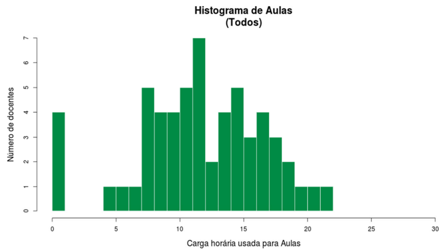
Figura 145 Histograma Aulas Todos
