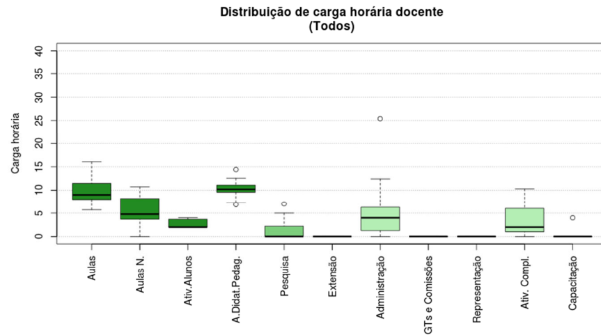
Figura 131 Boxplot Todos
