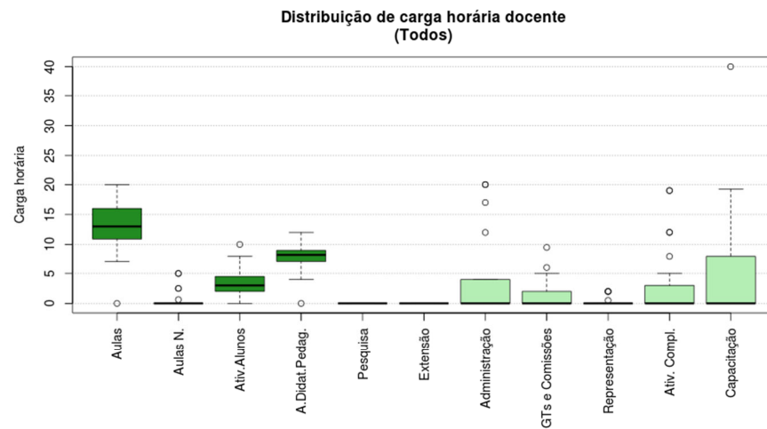
Figura 215 Boxplot Todos
