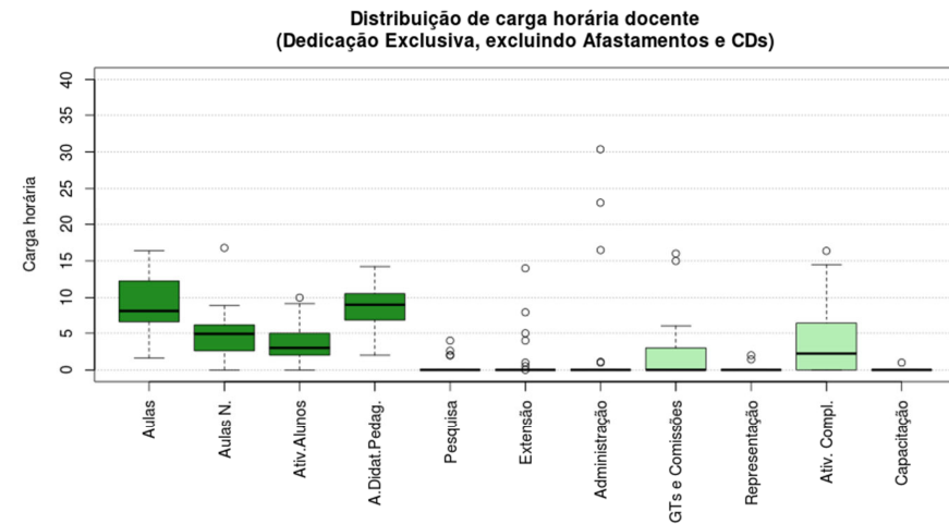
Figura 170 Boxplot Dedicação Exclusiva, excluindo Afastamentos e CDs
