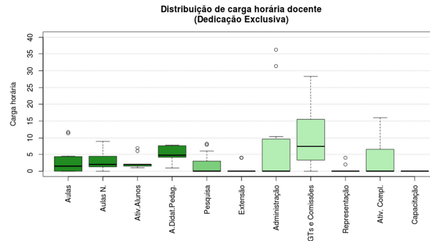
Figura 195 Boxplot Dedicação Exclusiva
