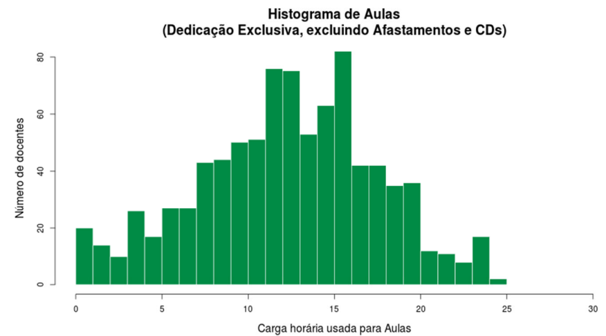
Figura 139 Histograma Aulas Dedicação Exclusiva excl. Afastamentos e CDs
