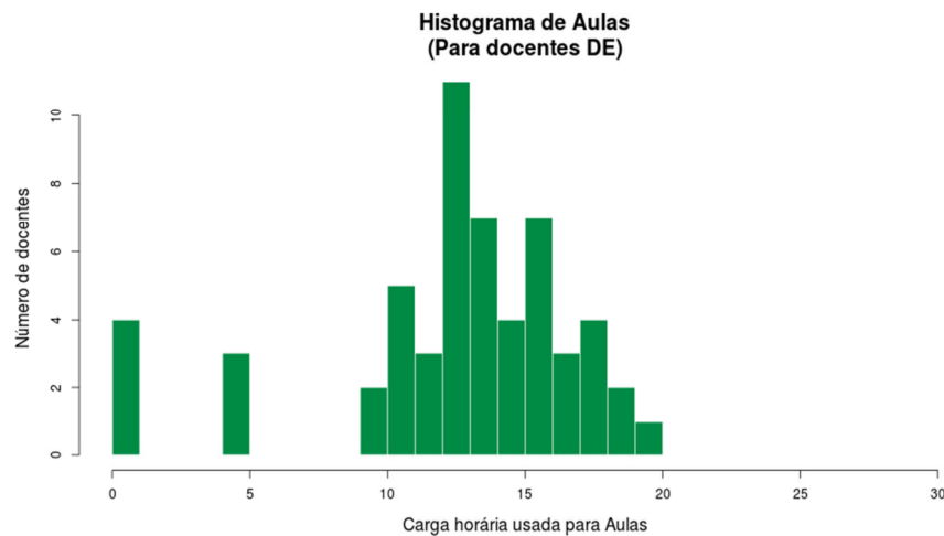
Figura 97 Histograma Aulas Dedicação Exclusiva
