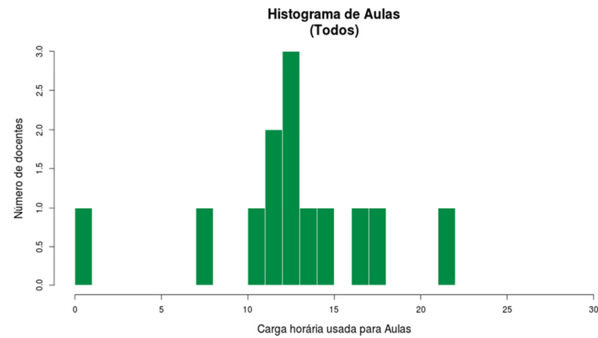
Figura 274 Histograma Aulas Todos
