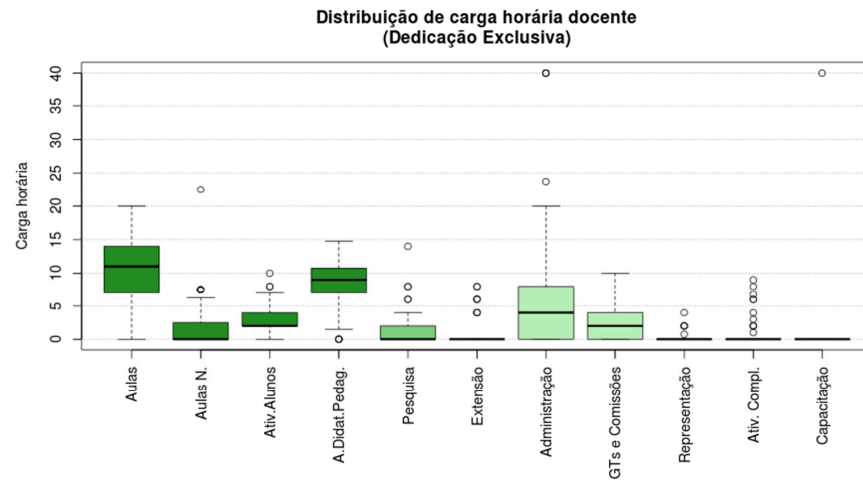
Figura 12 Boxplot Dedicação Exclusiva
