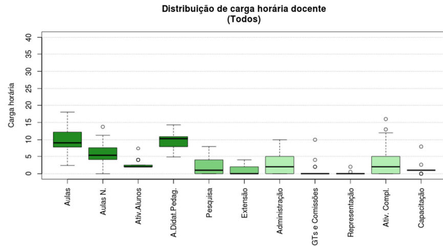
Figura 123 Boxplot Todos
