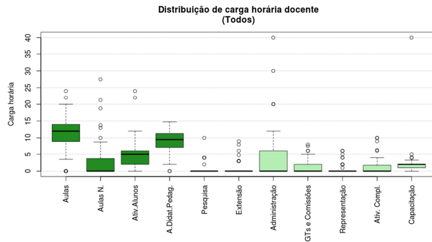
Figura 84 Boxplot Todos
