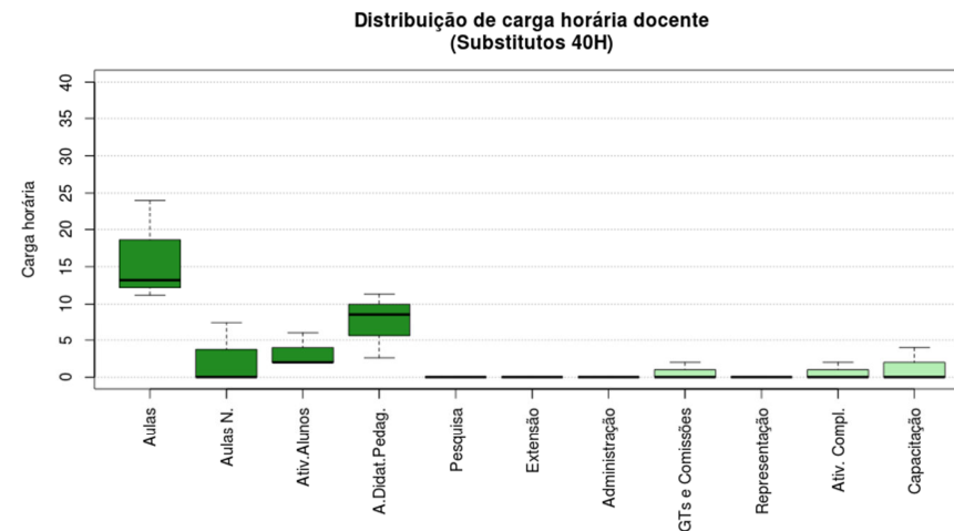
Figura 156 Boxplot Substitutos 40H
