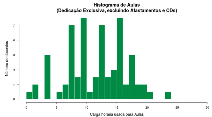
Figura 259 Histograma Aulas Dedicação Exclusiva excl. Afastamentos e CDs
