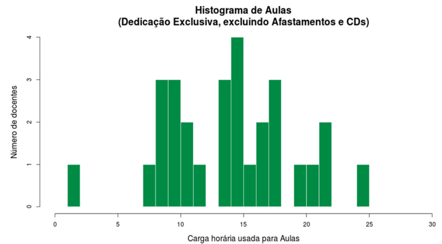
Figura 175 Histograma Aulas Dedicação Exclusiva excl. Afastamentos e CDs
