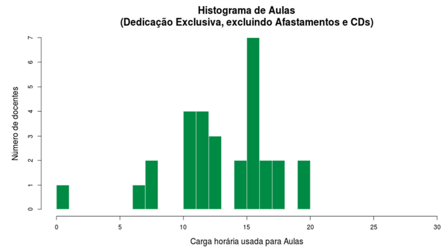
Figura 221 Histograma Aulas Dedicação Exclusiva excl. Afastamentos e CDs
