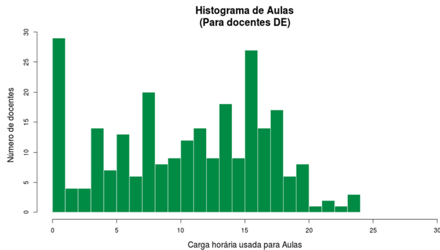
Figura 55 Histograma Aulas Dedicação Exclusiva
