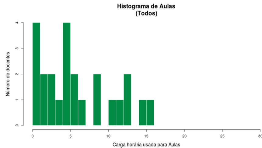
Figura 211 Histograma Aulas Todos
