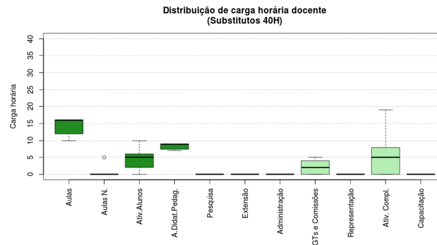
Figura 218 Boxplot Substitutos 40H
