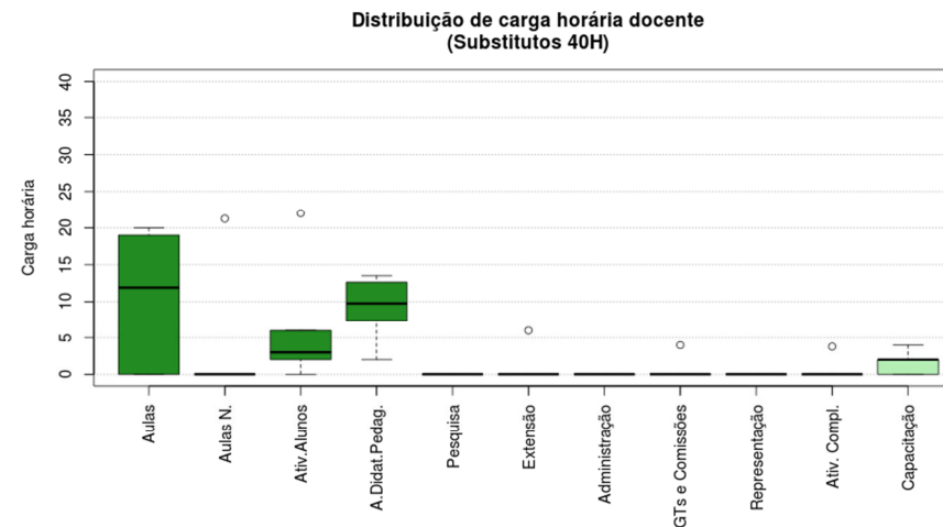
Figura 87 Boxplot Substitutos 40H
