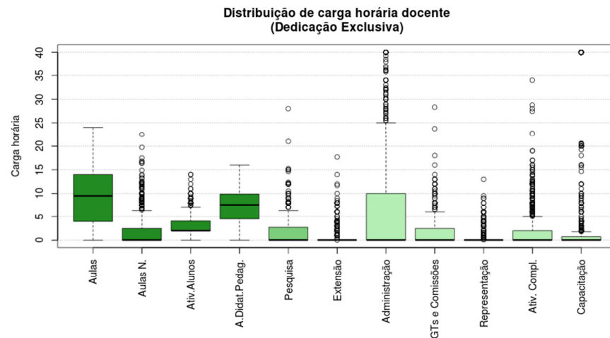
Figura 135 Boxplot Dedicação Exclusiva
