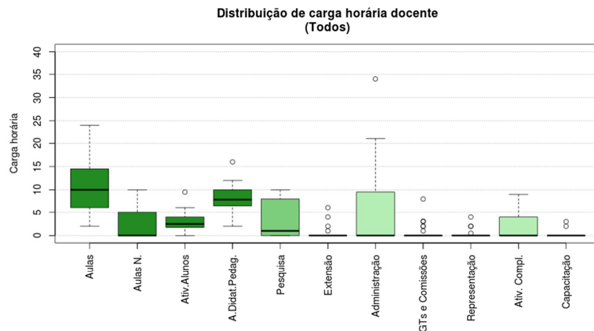
Figura 64 Boxplot Todos
