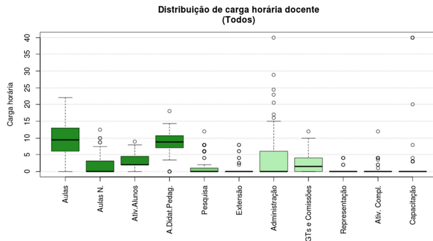
Figura 141 Boxplot Todos
