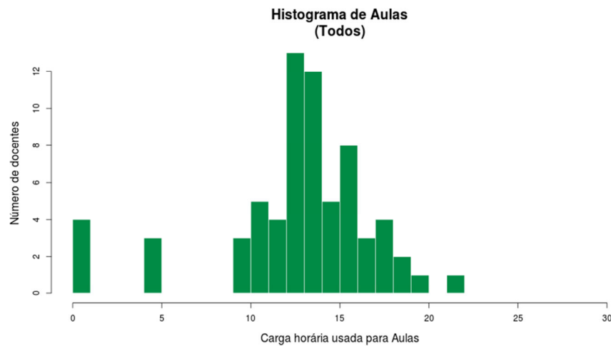
Figura 96 Histograma Aulas Todos
