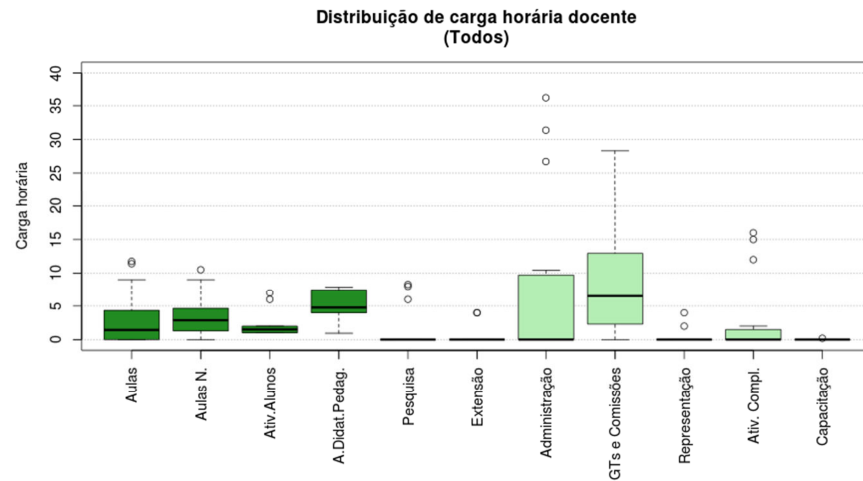
Figura 193 Boxplot Todos
