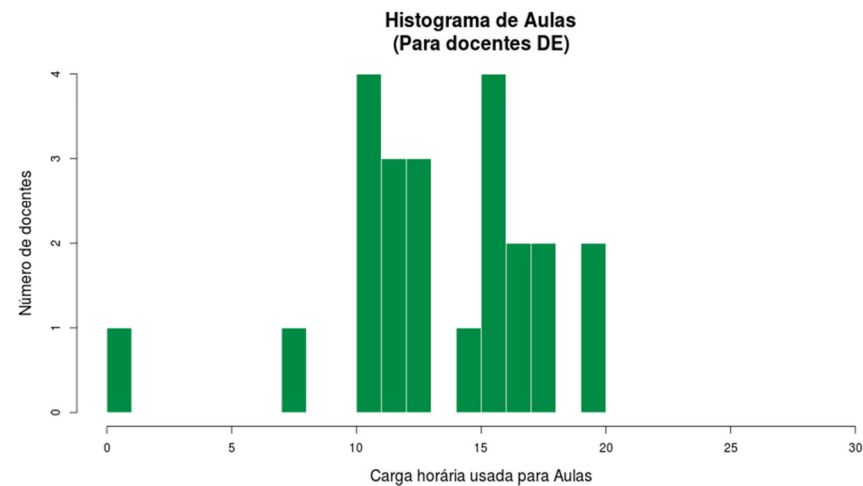
Figura 220 Histograma Aulas Dedicação Exclusiva
