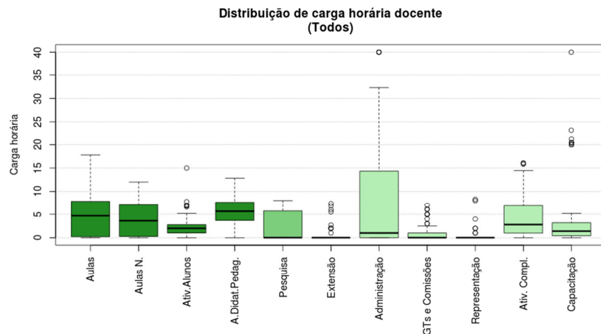
Figura 42 Boxplot Todos
