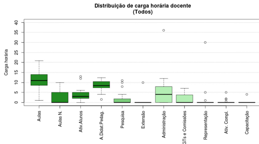
Figura 20 Boxplot Todos
