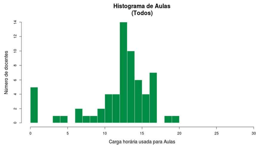
Figura 235 Histograma Aulas Todos
