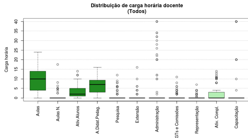
Figura 253 Boxplot Todos
