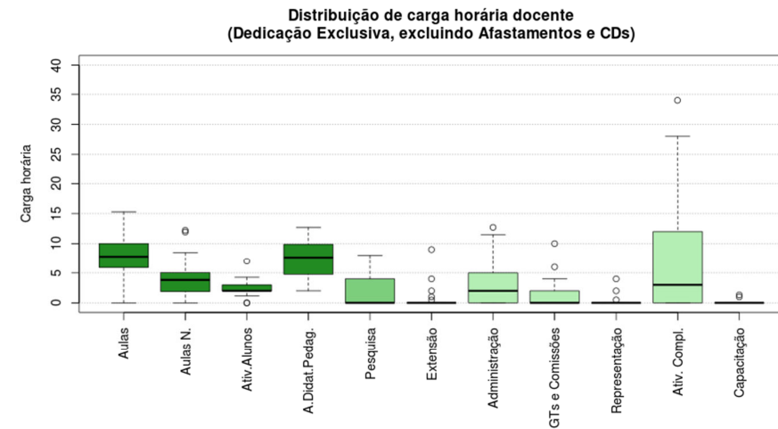
Figura 262 Boxplot Todos
