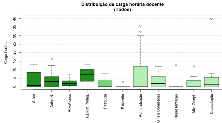
Figura 245 Boxplot Todos
