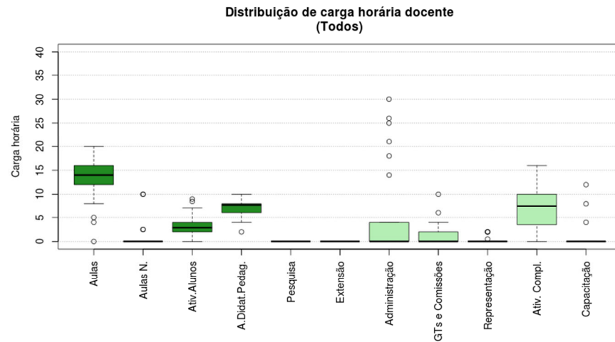
Figura 76 Boxplot Todos
