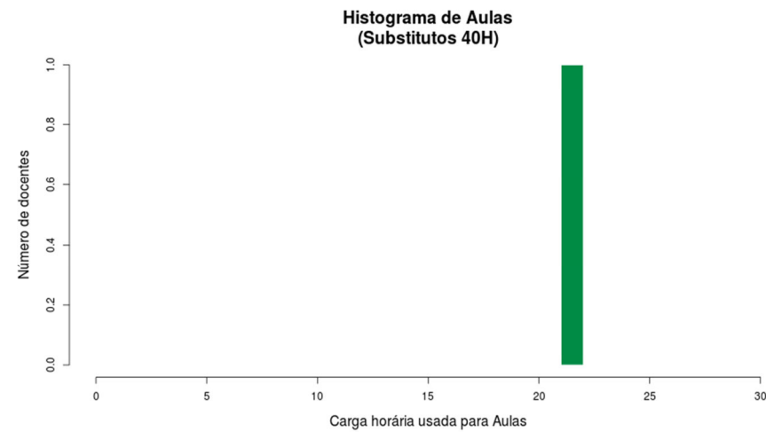
Figura 130 Histograma Aulas Substitutos 40H
