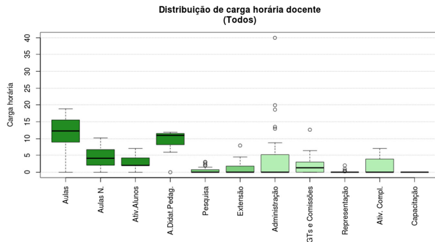
Figura 34 Boxplot Todos
