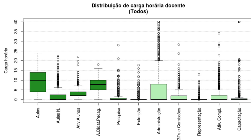
Figura 133 Boxplot Todos
