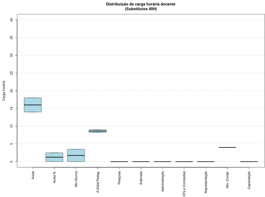
Figura 46: Boxplot Docentes Substitutos 40H
