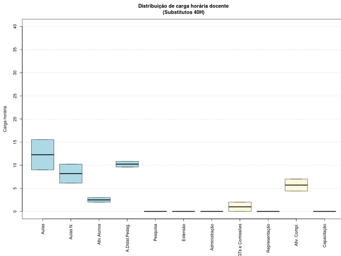
Figura 64: Boxplot Docentes Substitutos 40H
