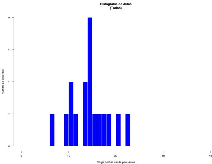
Figura 170: Histograma Aulas Todos os Docentes
