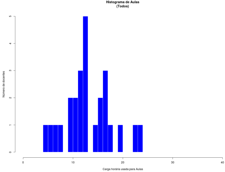
Figura 100: Histograma Aulas Todos os Docentes
