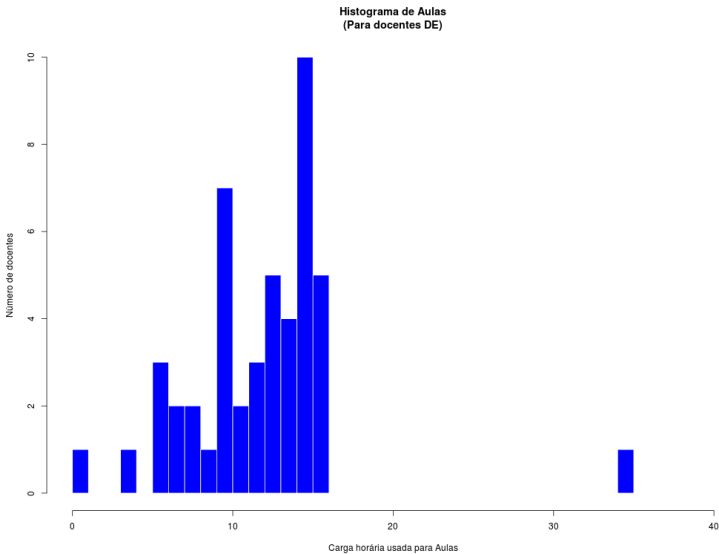
Figura 57: Histograma Aulas para Docentes DE
