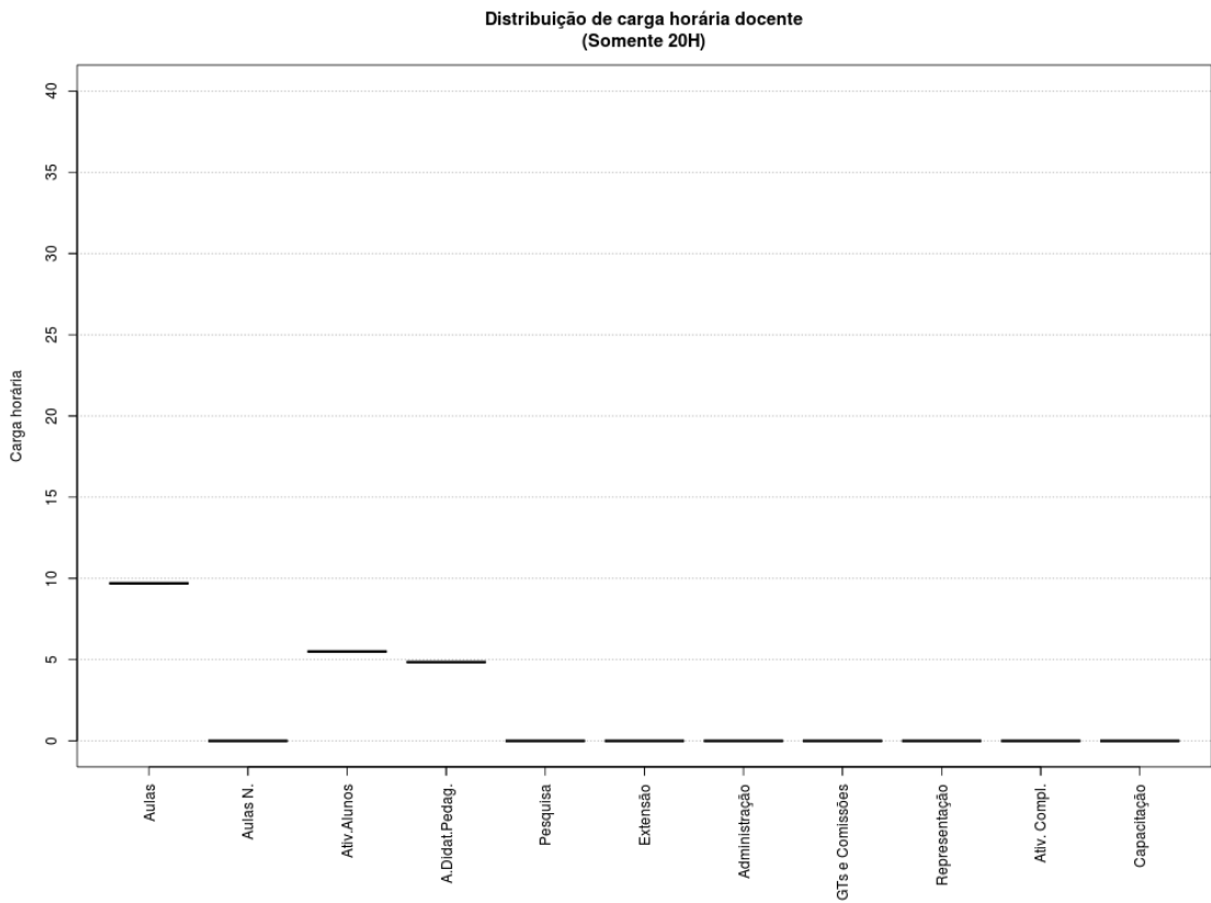
Figura 38: Boxplot Docentes Todos 20H
