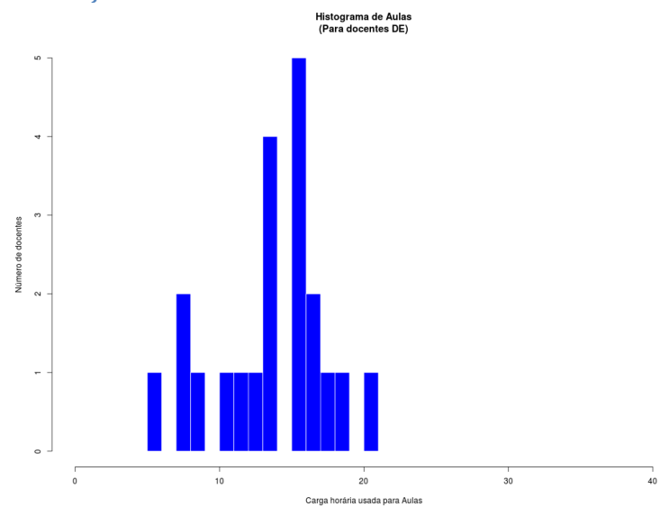
Figura 125: Histograma Aulas para Docentes DE
