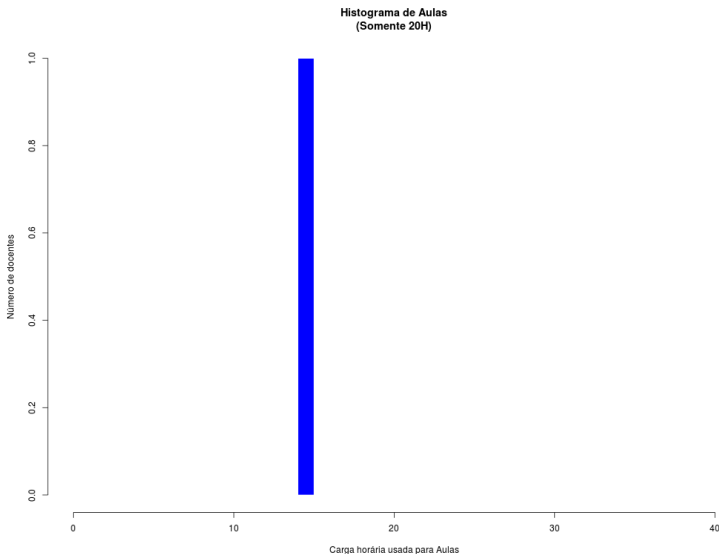
Figura 59: Histograma Aulas para Docentes 20H
