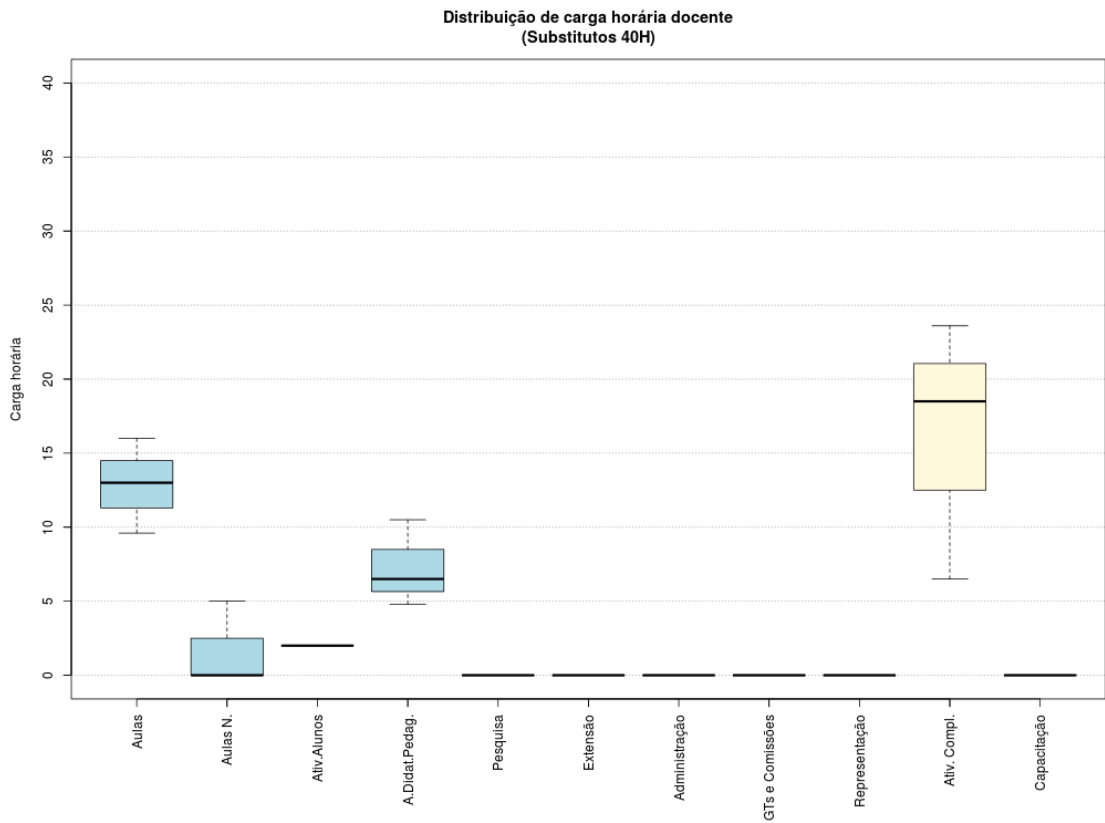
Figura 143: Boxplot Docentes Substitutos 40H
