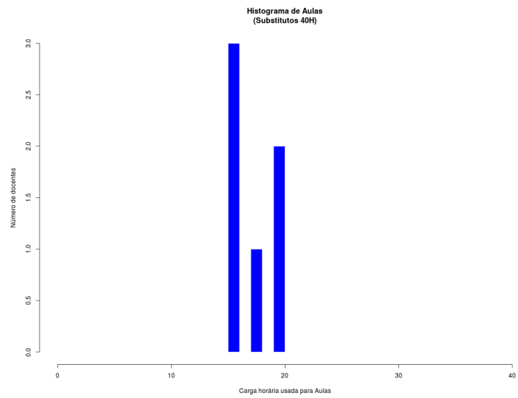
Figura 128: Histograma Aulas para Docentes Substitutos 40
