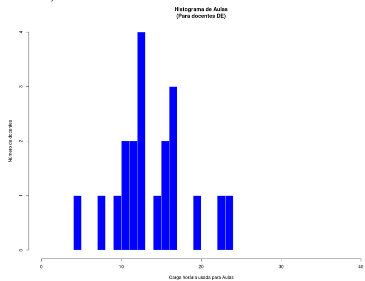
Figura 101: Histograma Aulas para Docentes DE
