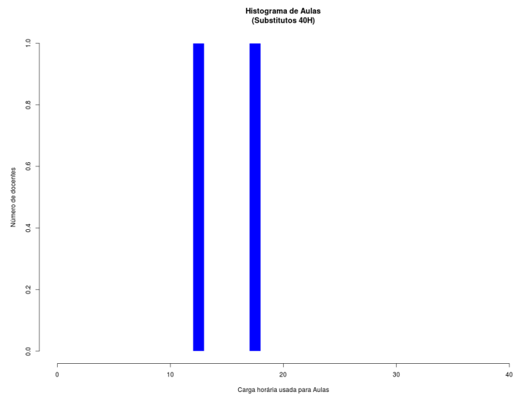
Figura 104: Histograma Aulas para Docentes Substitutos 40
