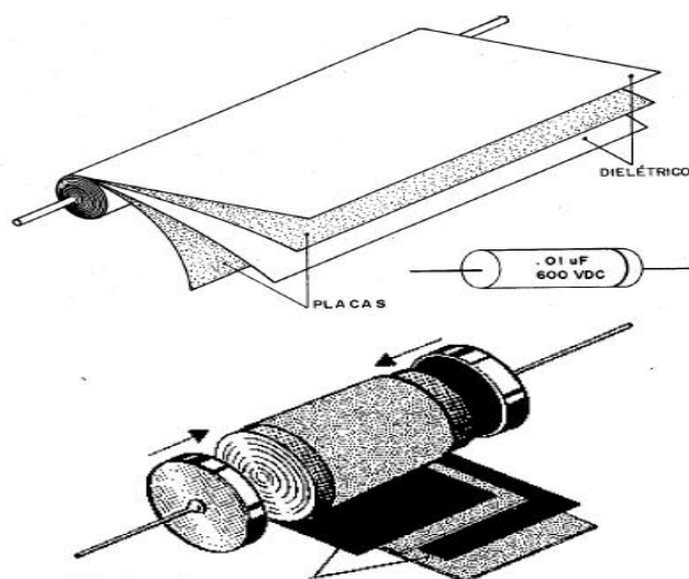
Figura – capacitor.
